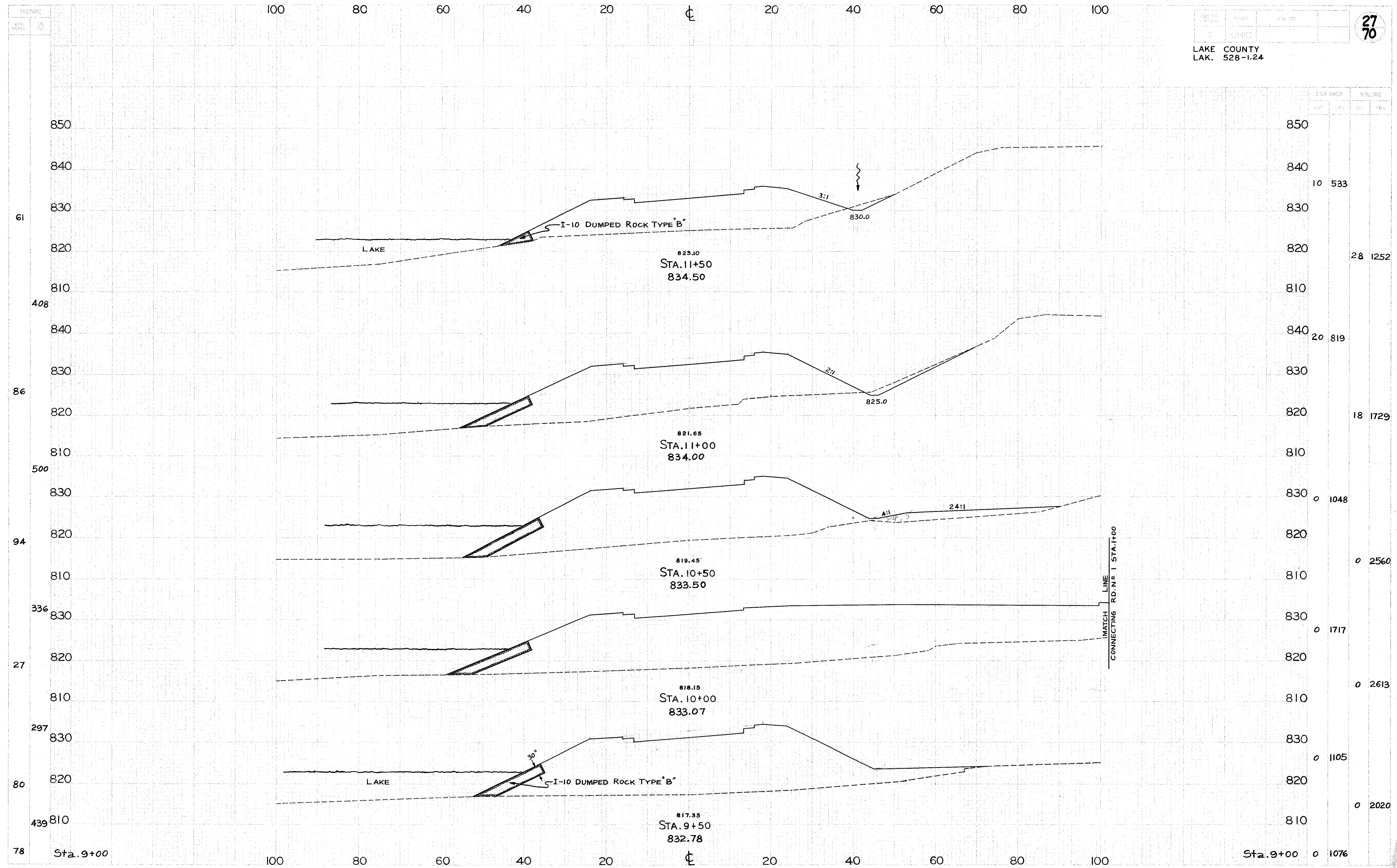
S.R. 528... CROSS SECTIONS... STA. 9+50 TO STA. 11+50
