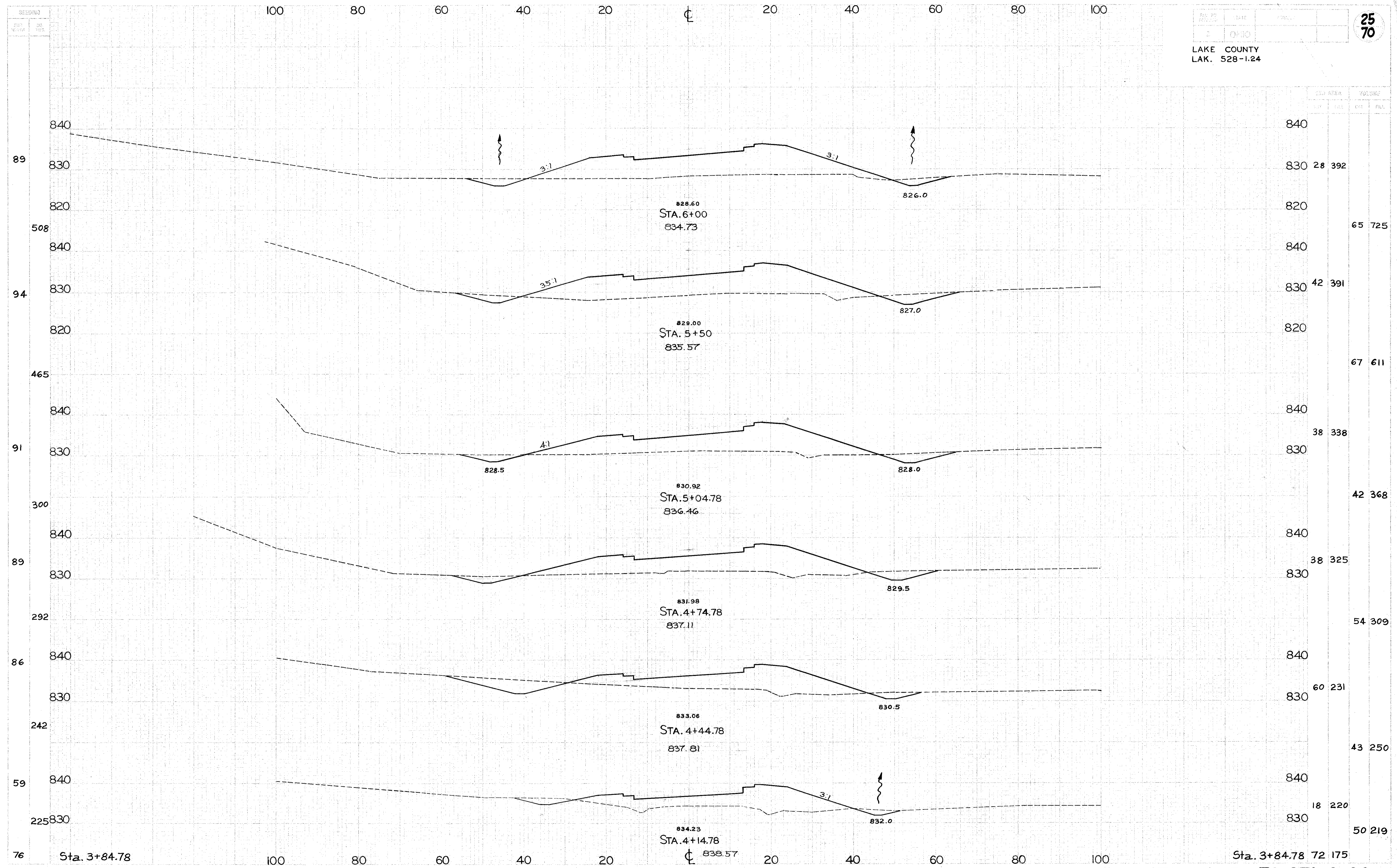
S.R. 528... CROSS SECTIONS... STA. 4+14.78 TO STA. 6+00
