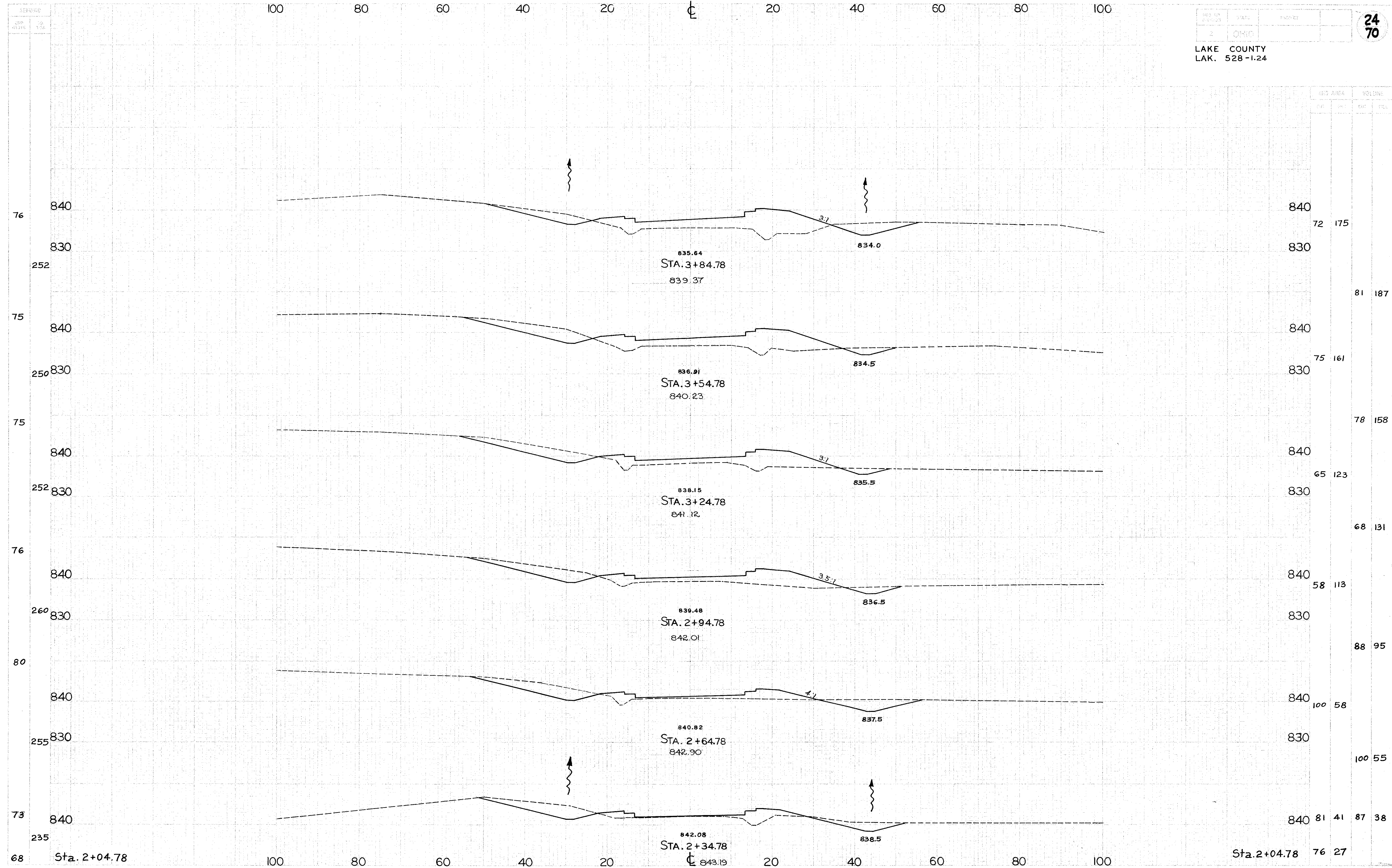
S.R. 528... CROSS SECTIONS ... STA. 2+34.78 TO STA. 3+84.78
