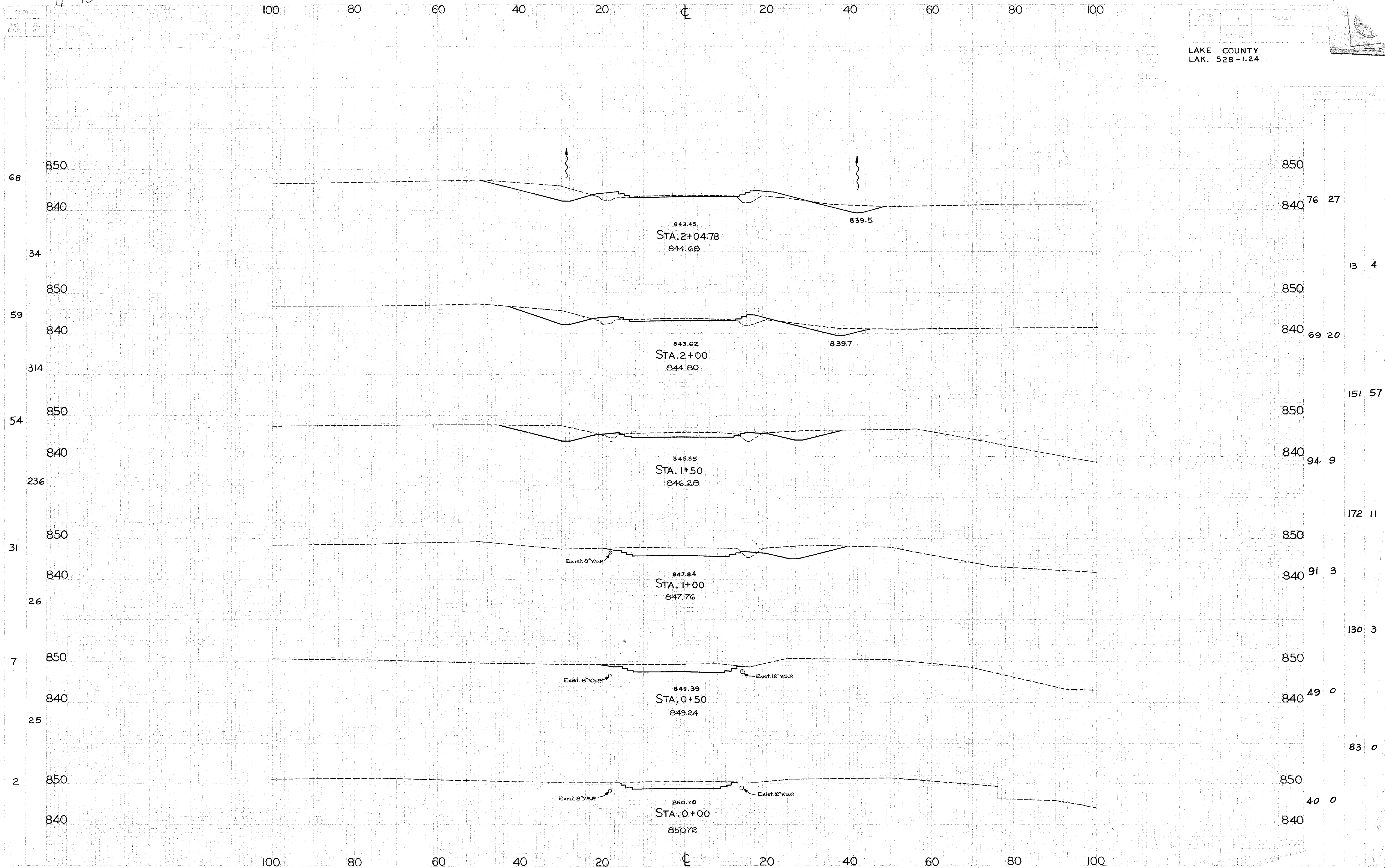
S.R. 528... CROSS SECTIONS... STA. 0+00 TO STA. 2+04.78
