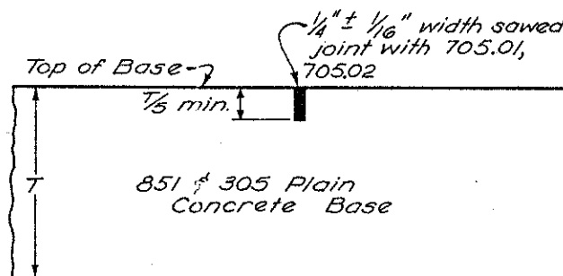
SECTION - 851 & 305 BASE
