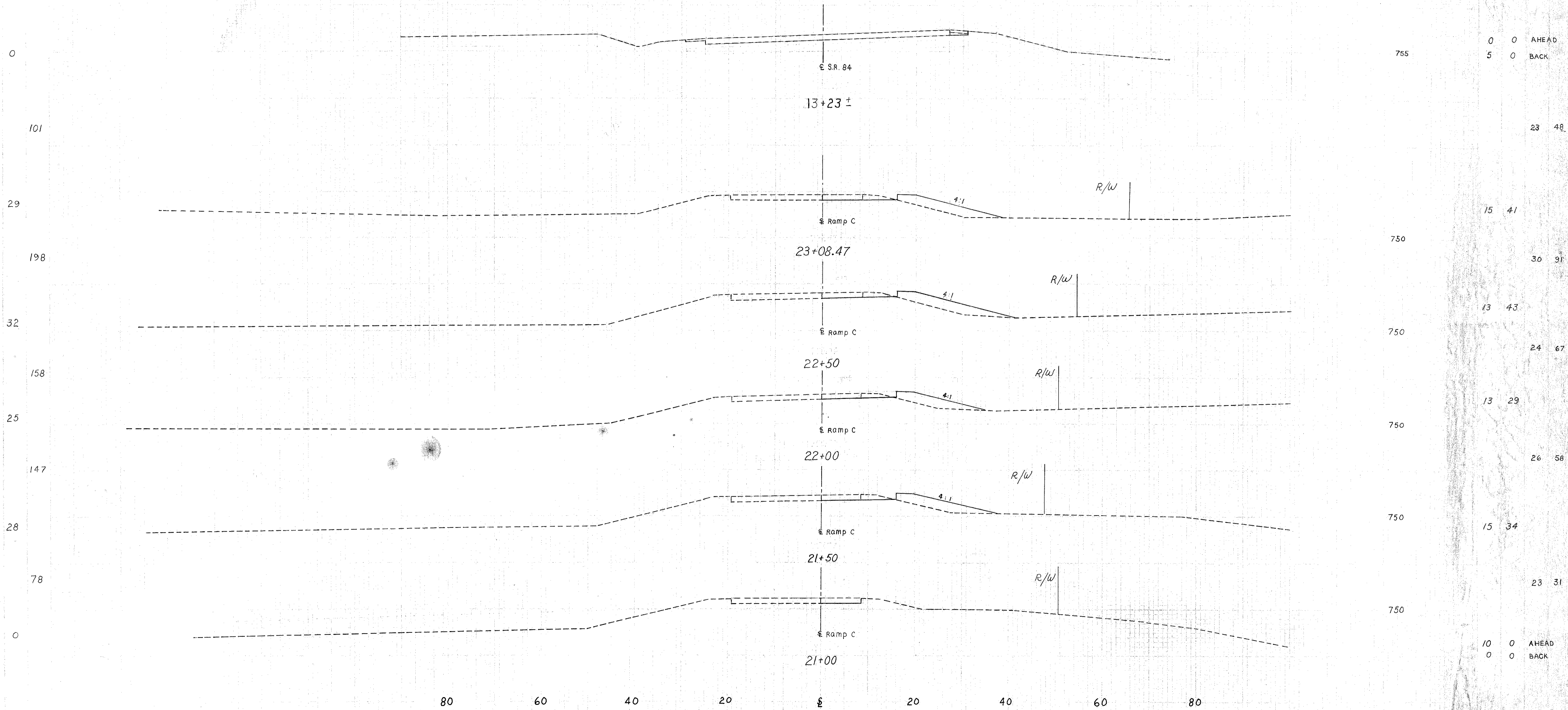
CROSS SECTIONS RAMP "C" STA. 21+00 TO STA. 13+23.1 (S.R. 84)
