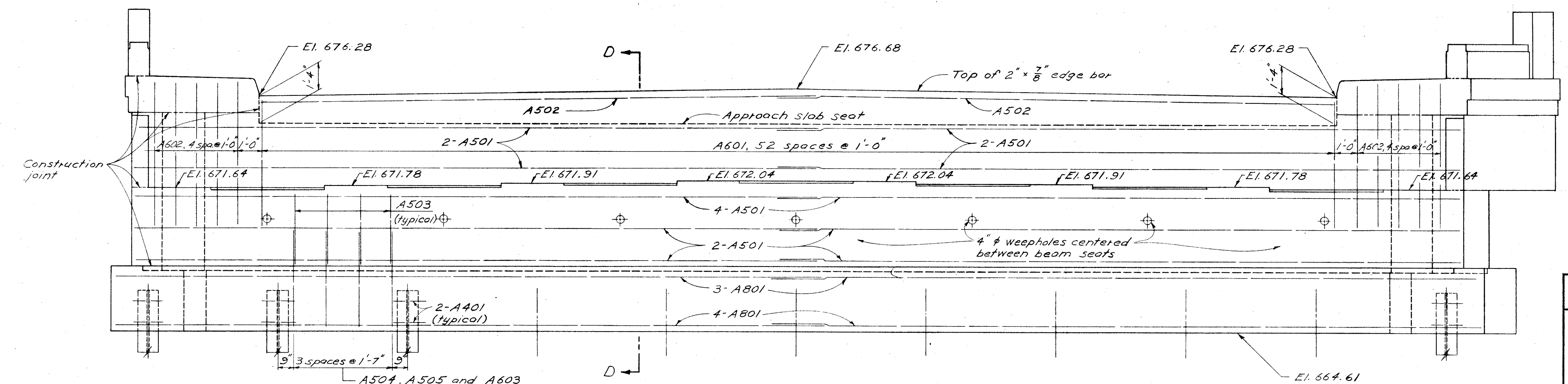
ELEVATION
