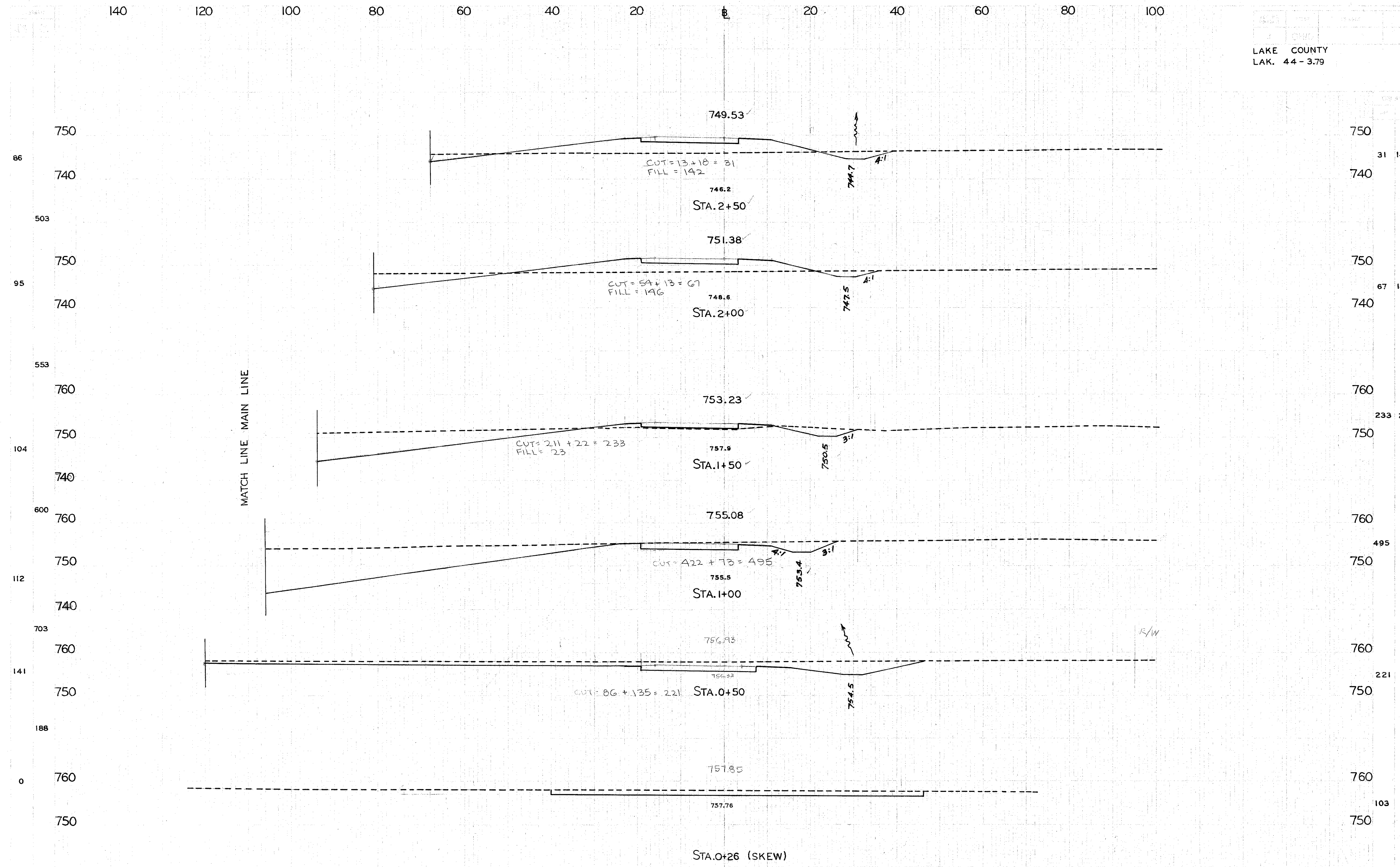
RAMP "B" STA. 0+26 TO STA. 2+50
