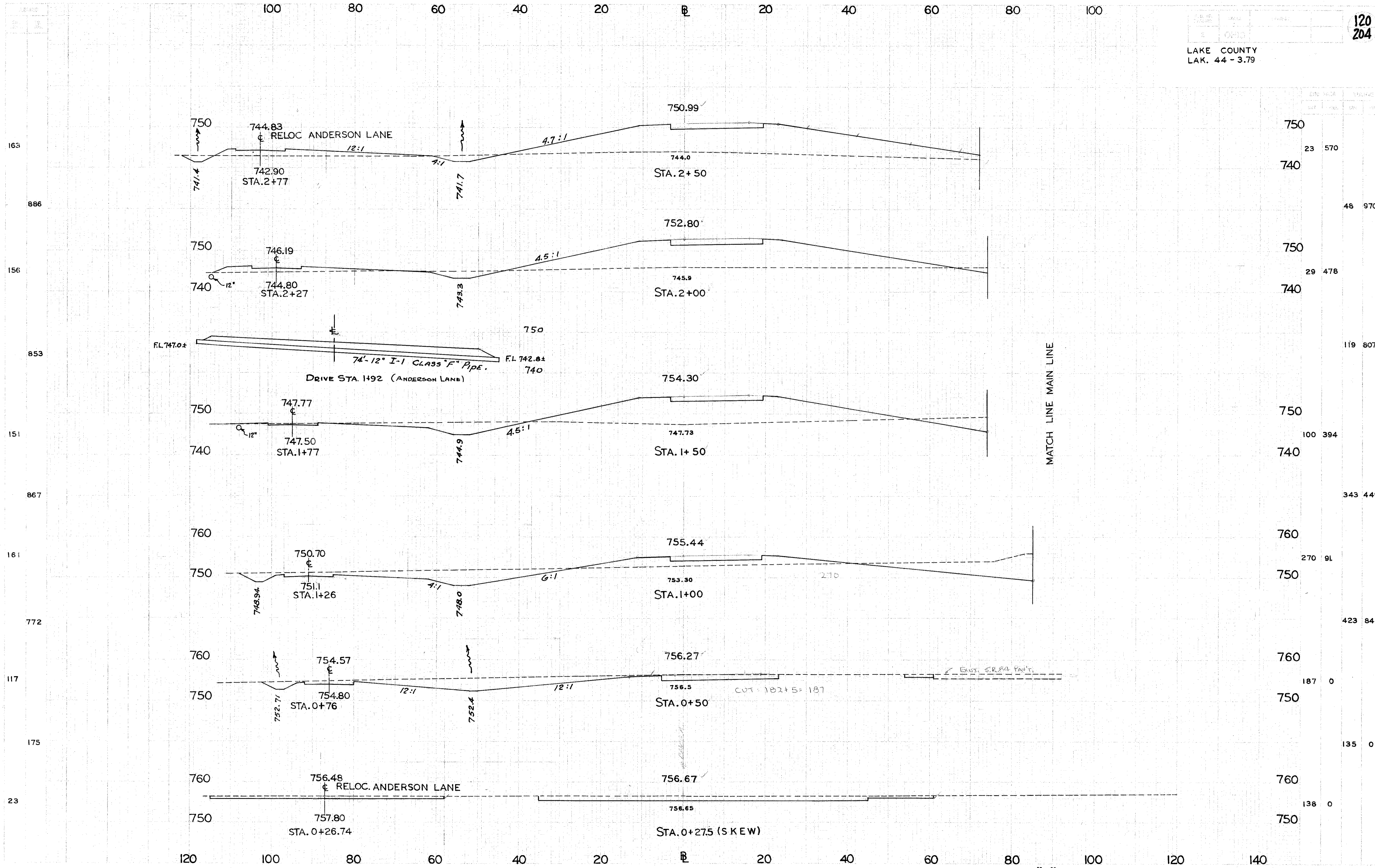
RAMP "A" STA. 0+27.5 TO STA. 2+50
