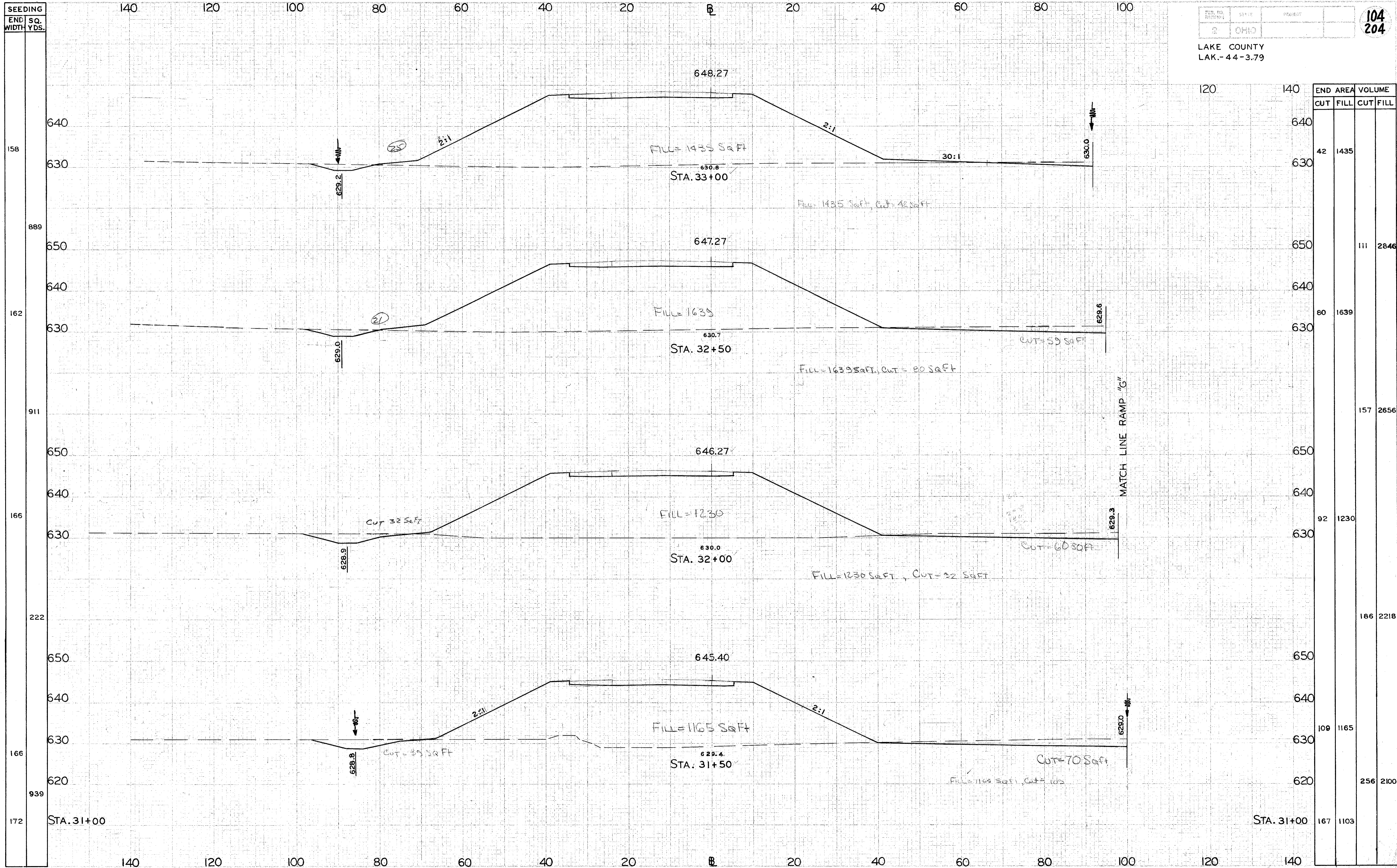
RAMP "E" STA. 31+50 TO STA. 33+00
