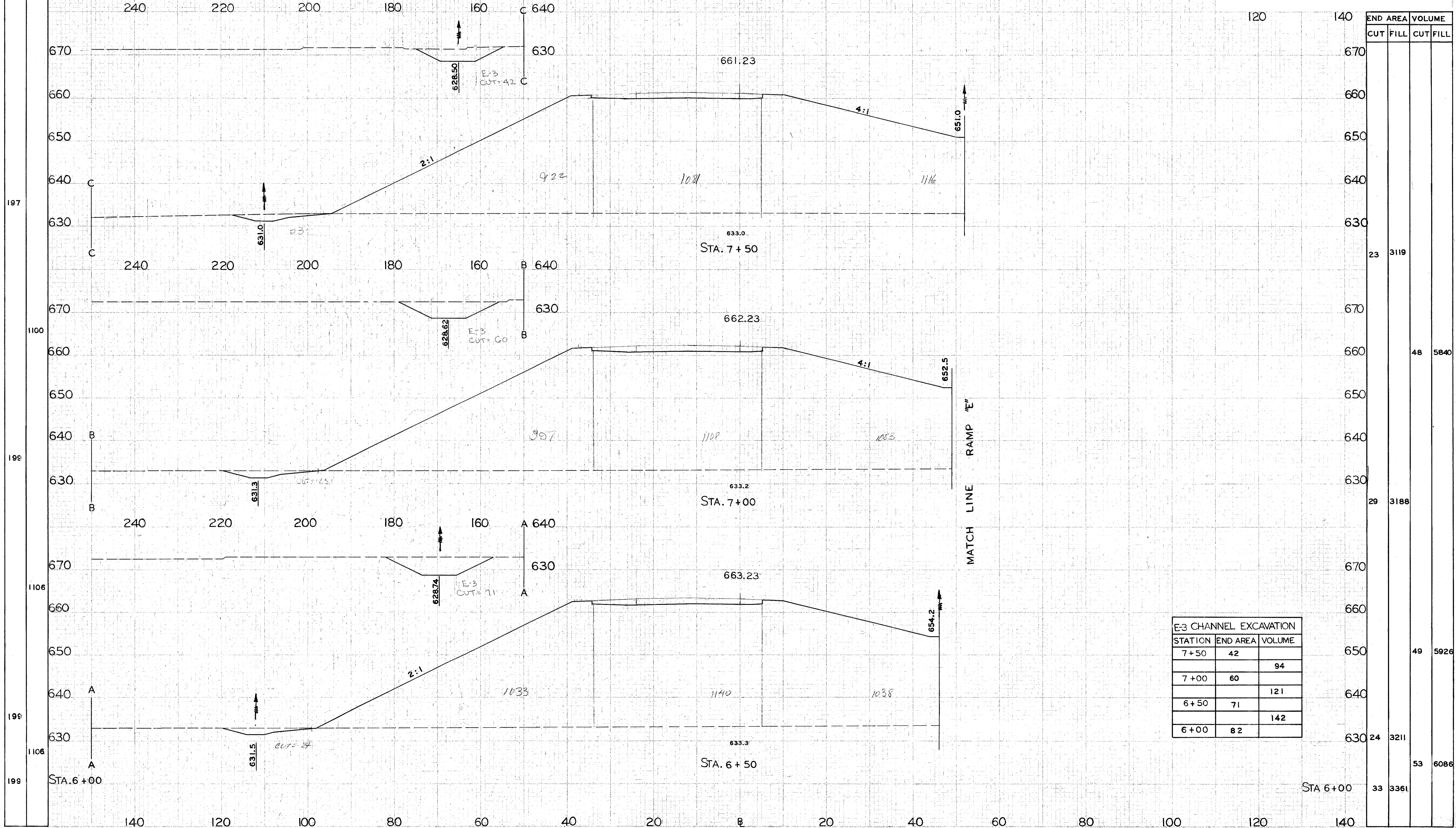
RAMP "G" STA. 6+50 TO STA. 7+50
