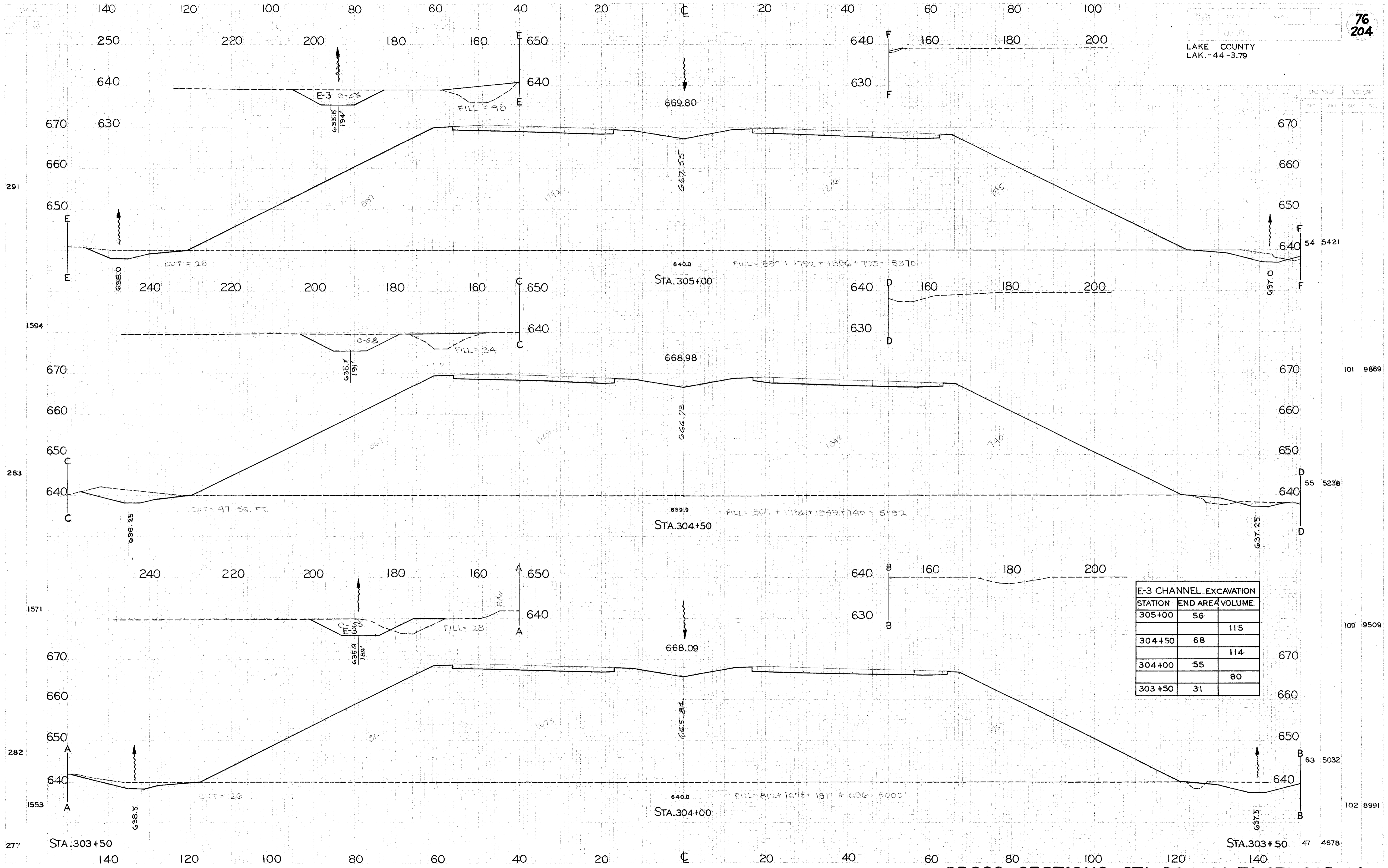
CROSS SECTIONS STA. 304+00 TO STA. 305+00
