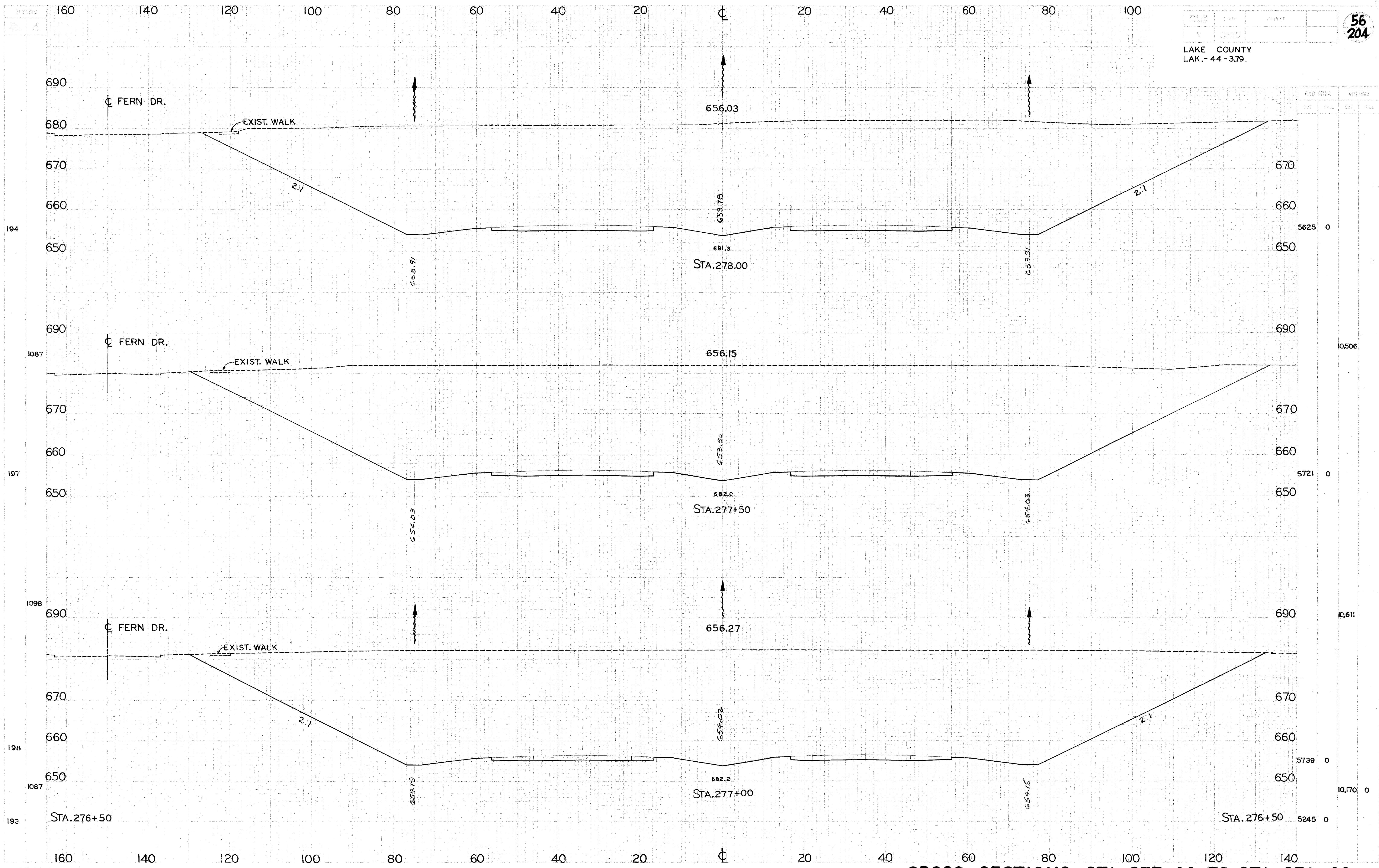
CROSS SECTIONS STA. 277+00 TO STA. 278+00
