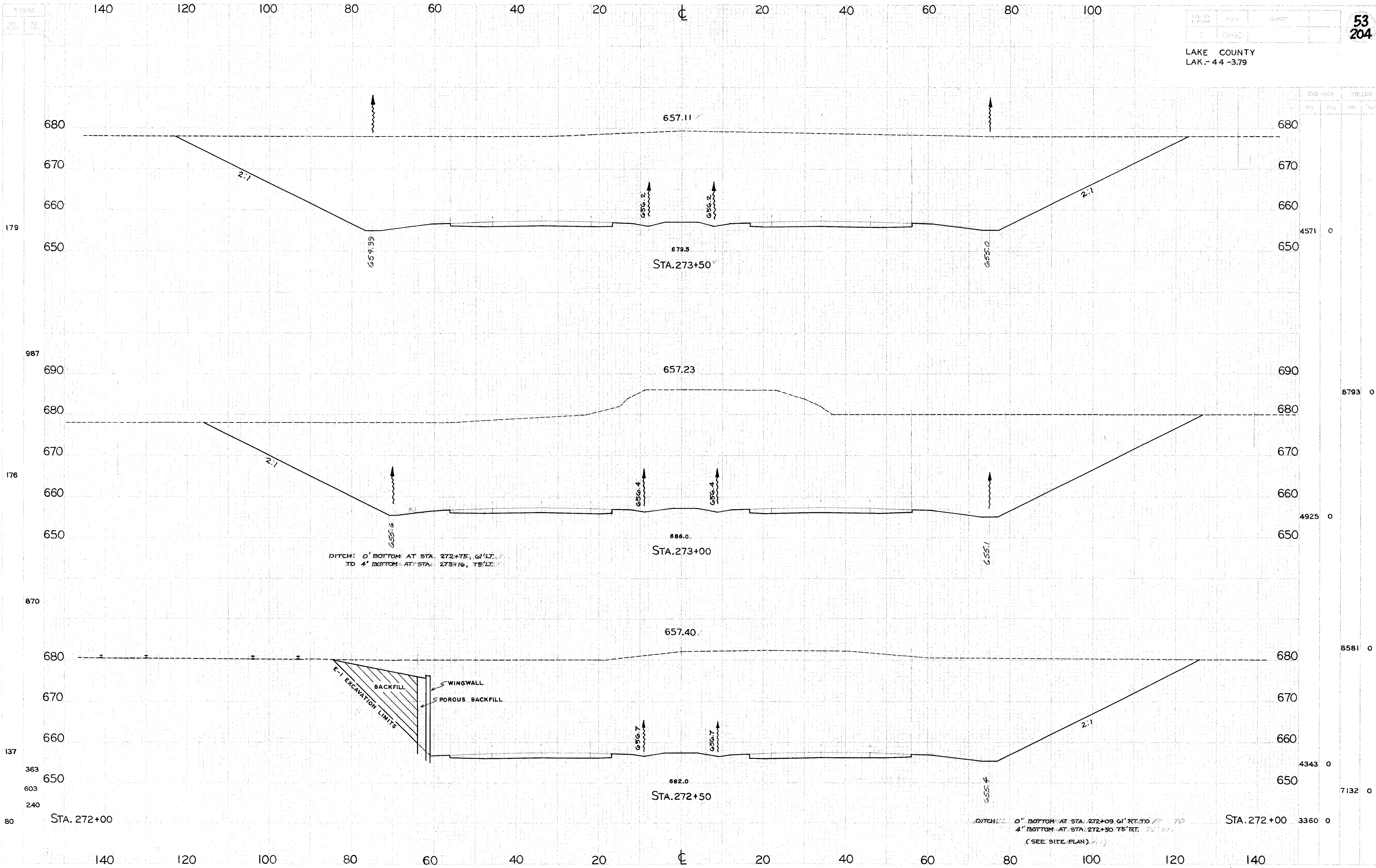
CROSS SECTIONS STA. 272+50 TO STA. 273+50
