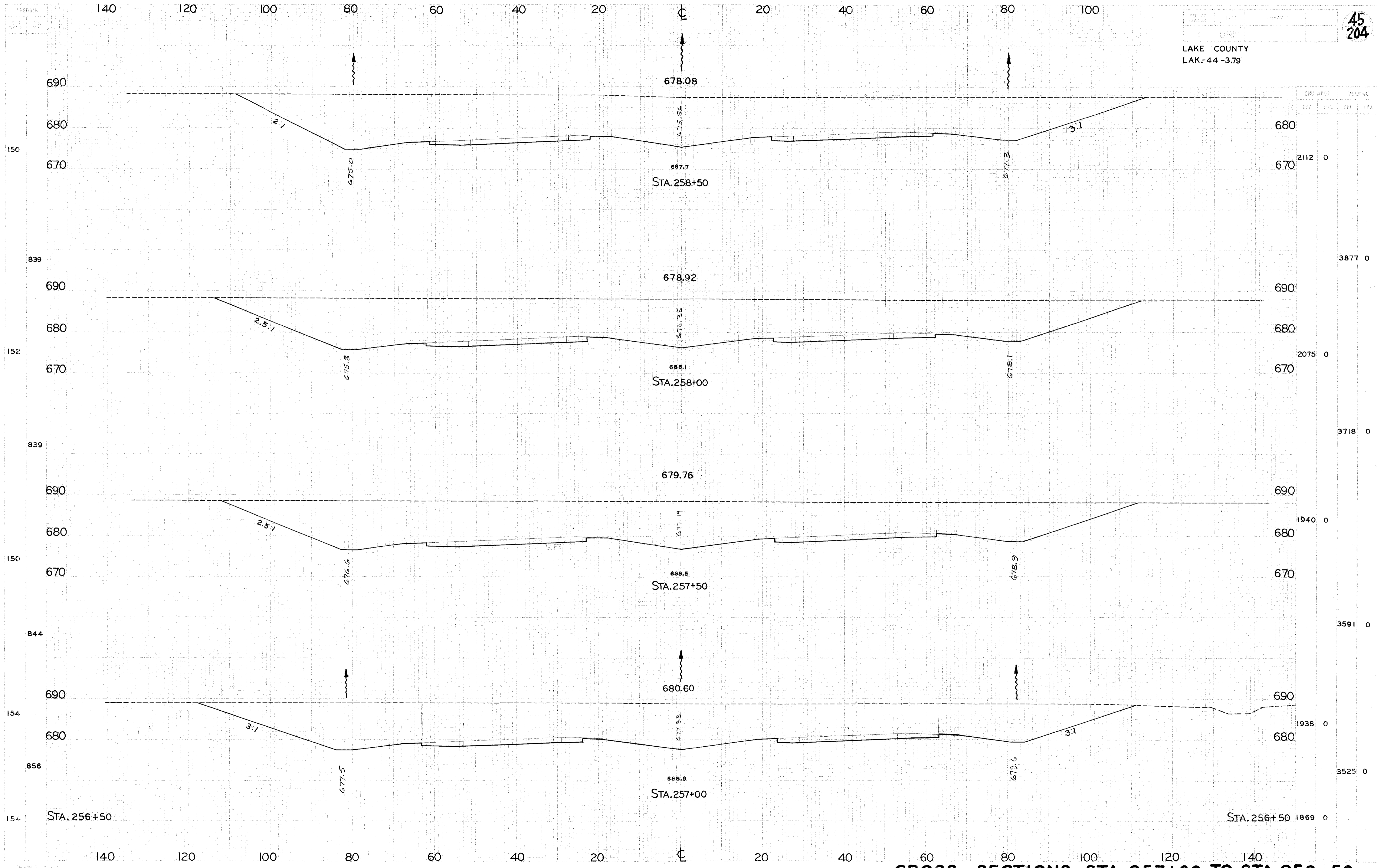
CROSS SECTIONS STA. 257+00 TO STA. 258+50
