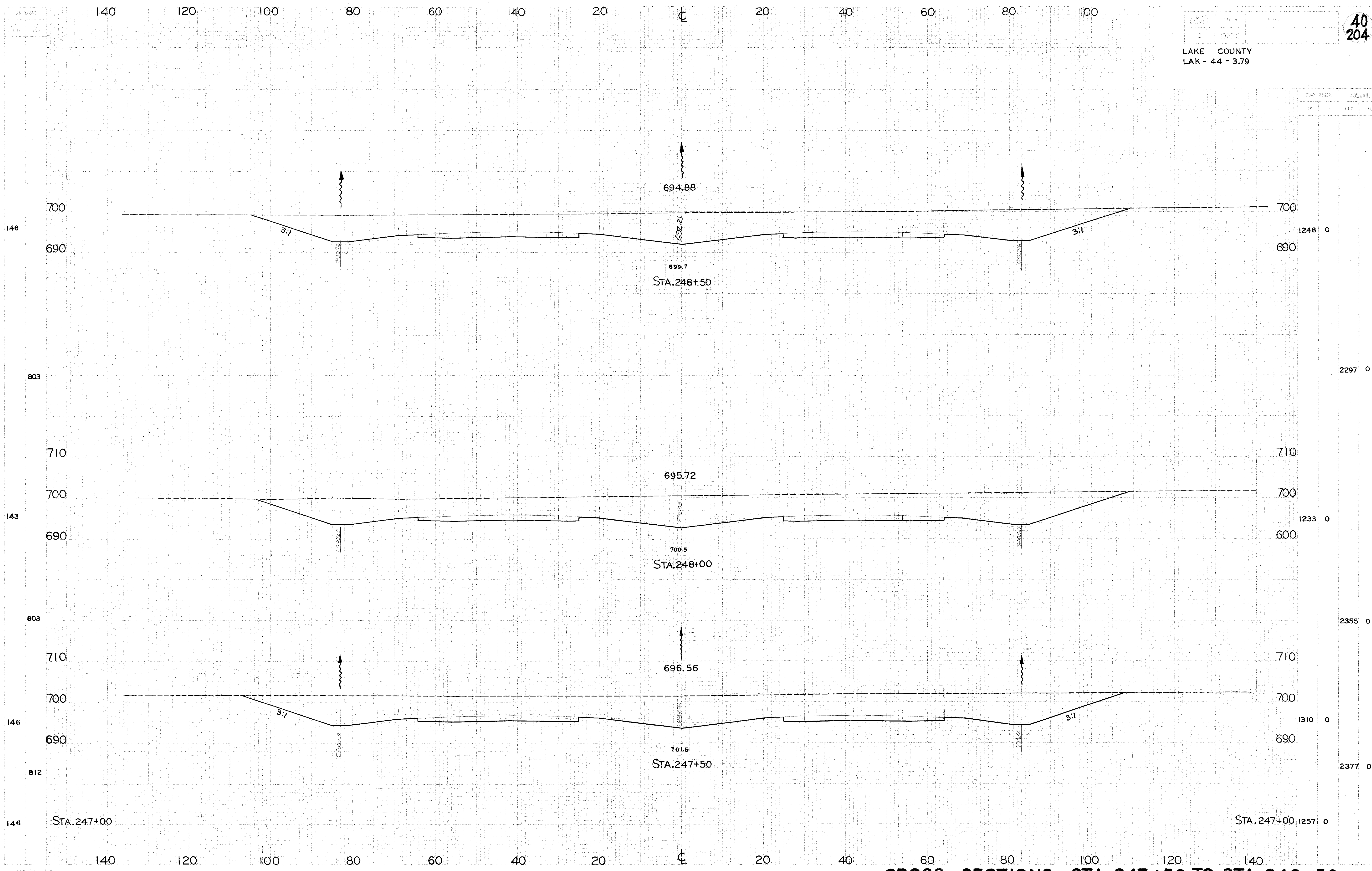
CROSS SECTIONS STA. 247+50 TO STA. 248+50
