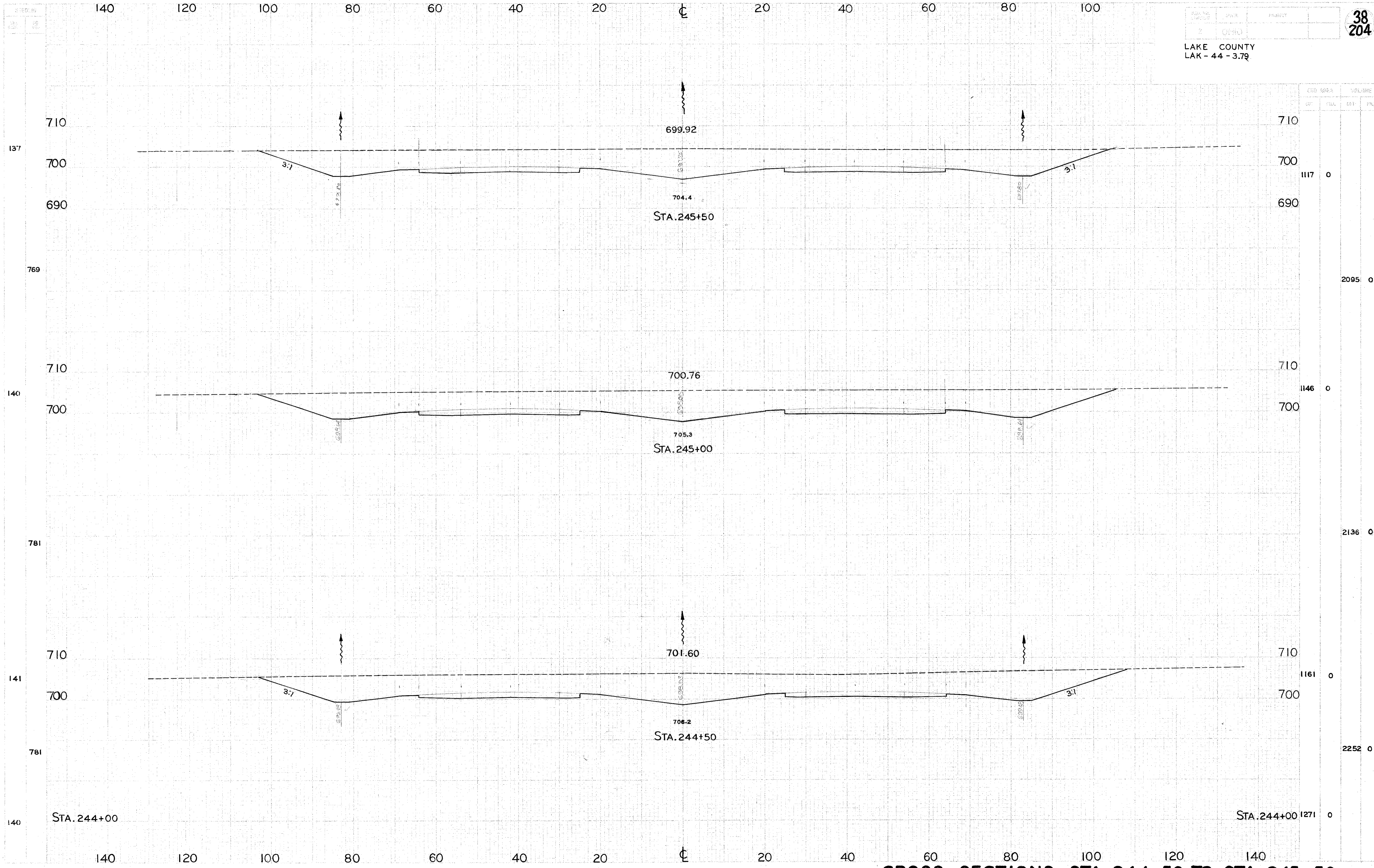
CROSS SECTIONS STA. 244+50 TO STA. 245+50
