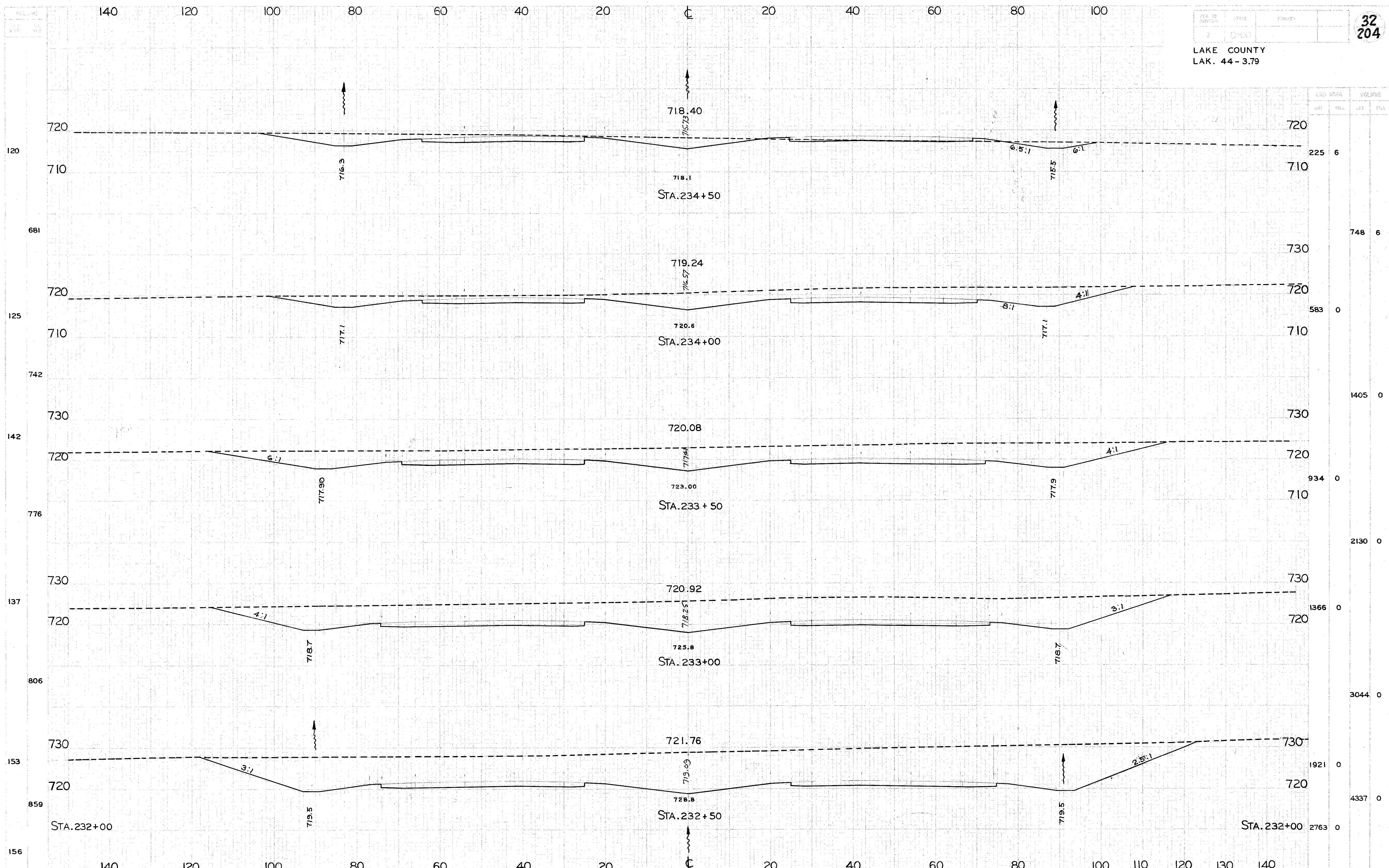
CROSS SECTIONS STA. 232+50 TO STA. 234+50
