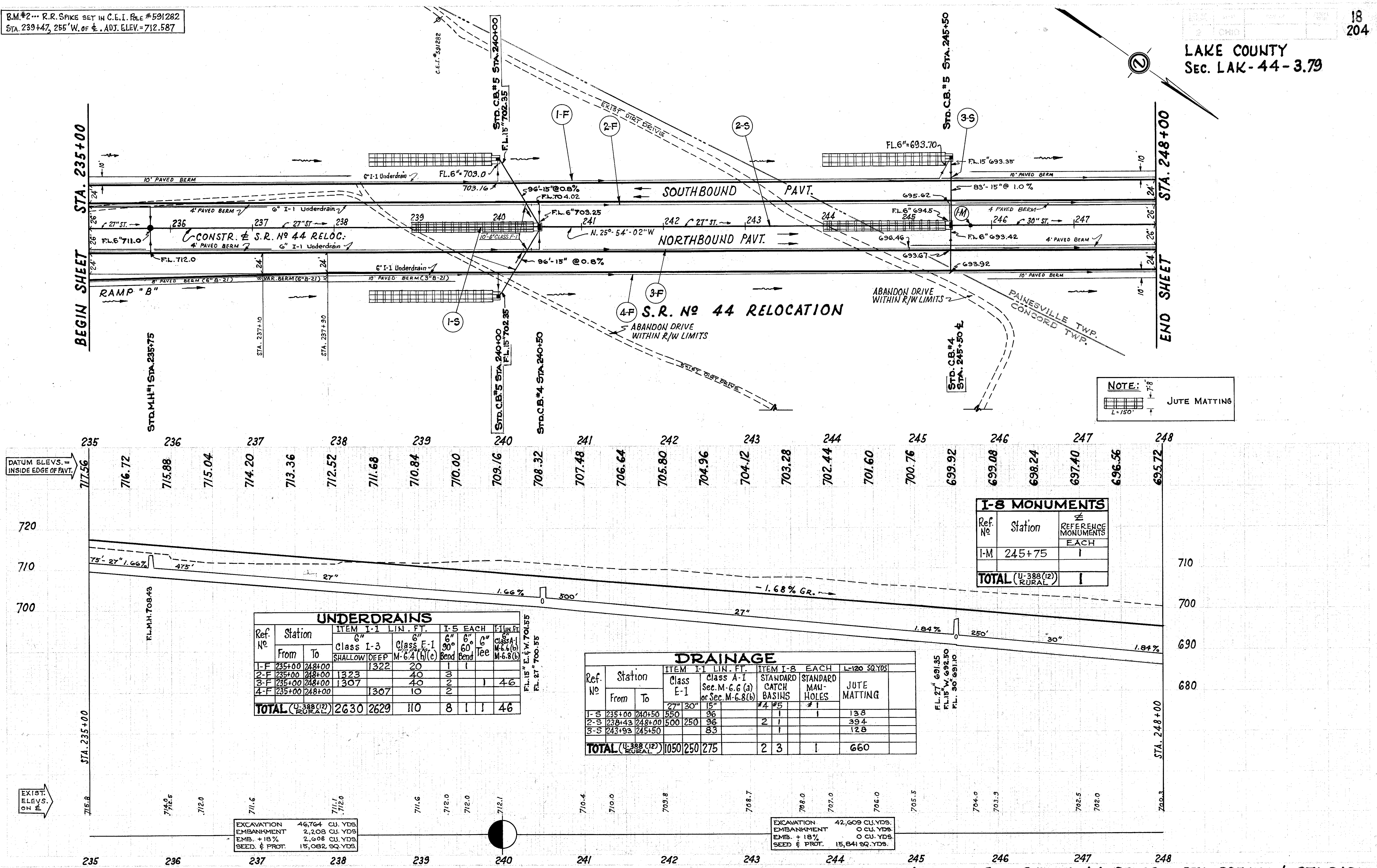
PLAN & PROFILE ... S.R. No 44 RELOC. ... STA. 235+00 to STA. 248+00
