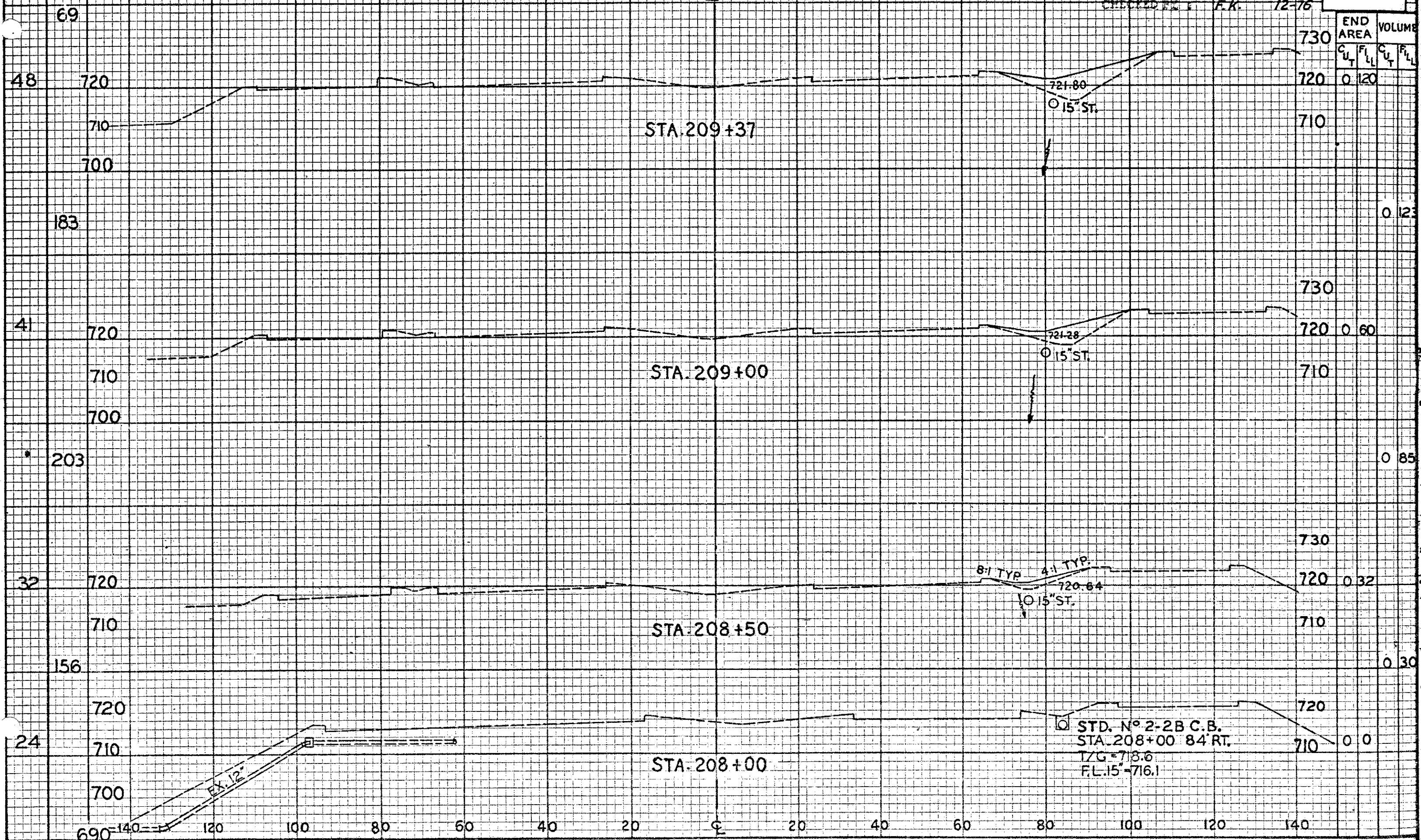
X-SECTIONS STA. 208+00 to STA. 209+37
