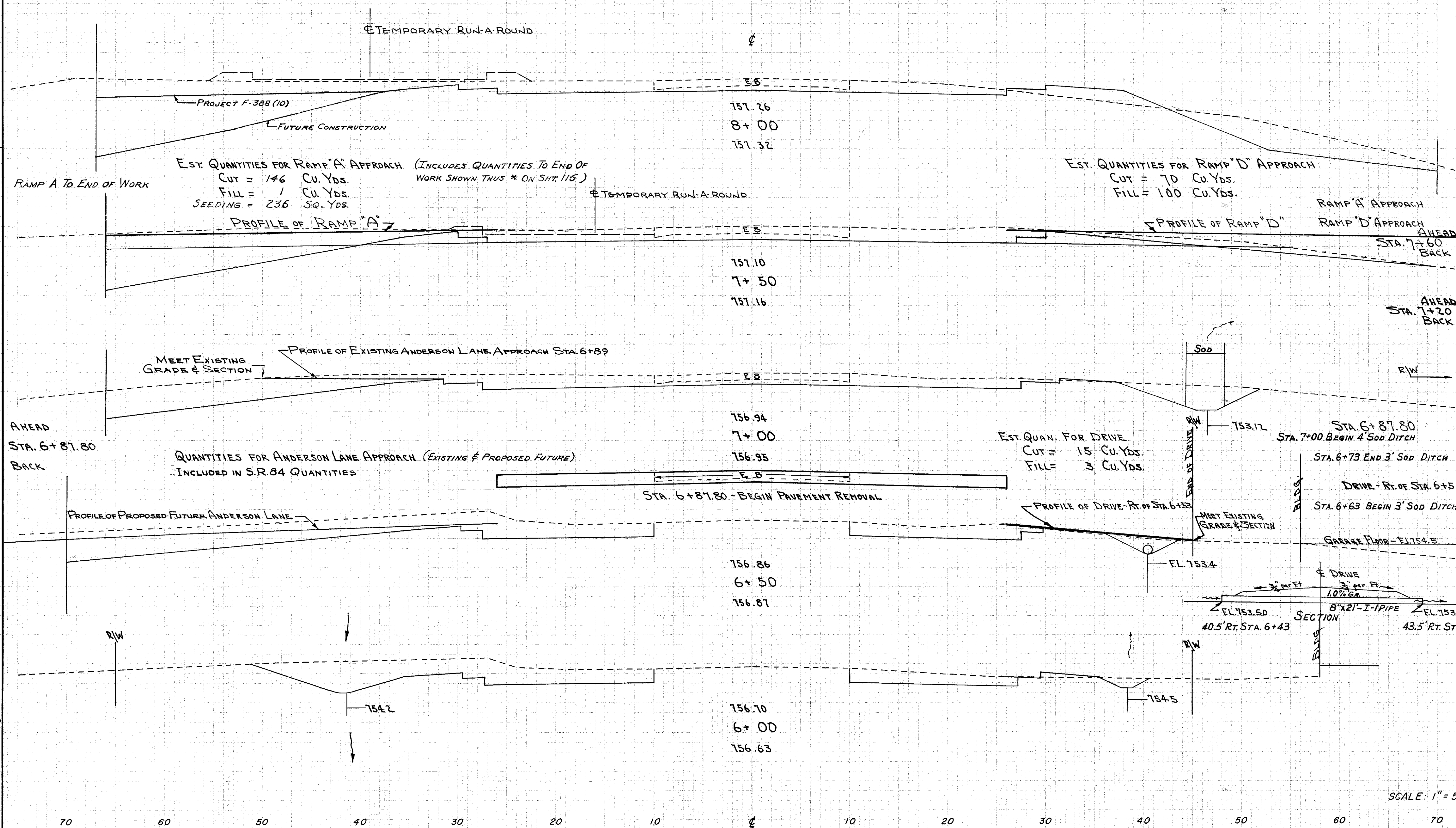
S.R. 84 STA. 6+00 TO STA. 8+00
