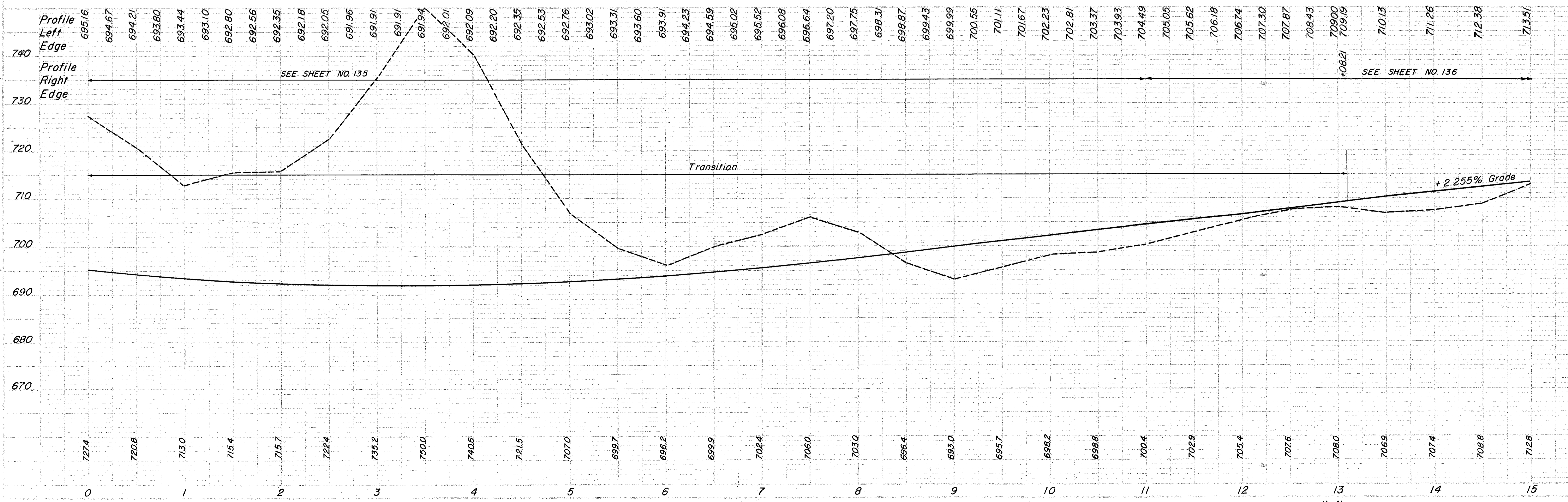
PLAN & PROFILE RAMP "D" STA. 0+00 TO STA. 15+00
