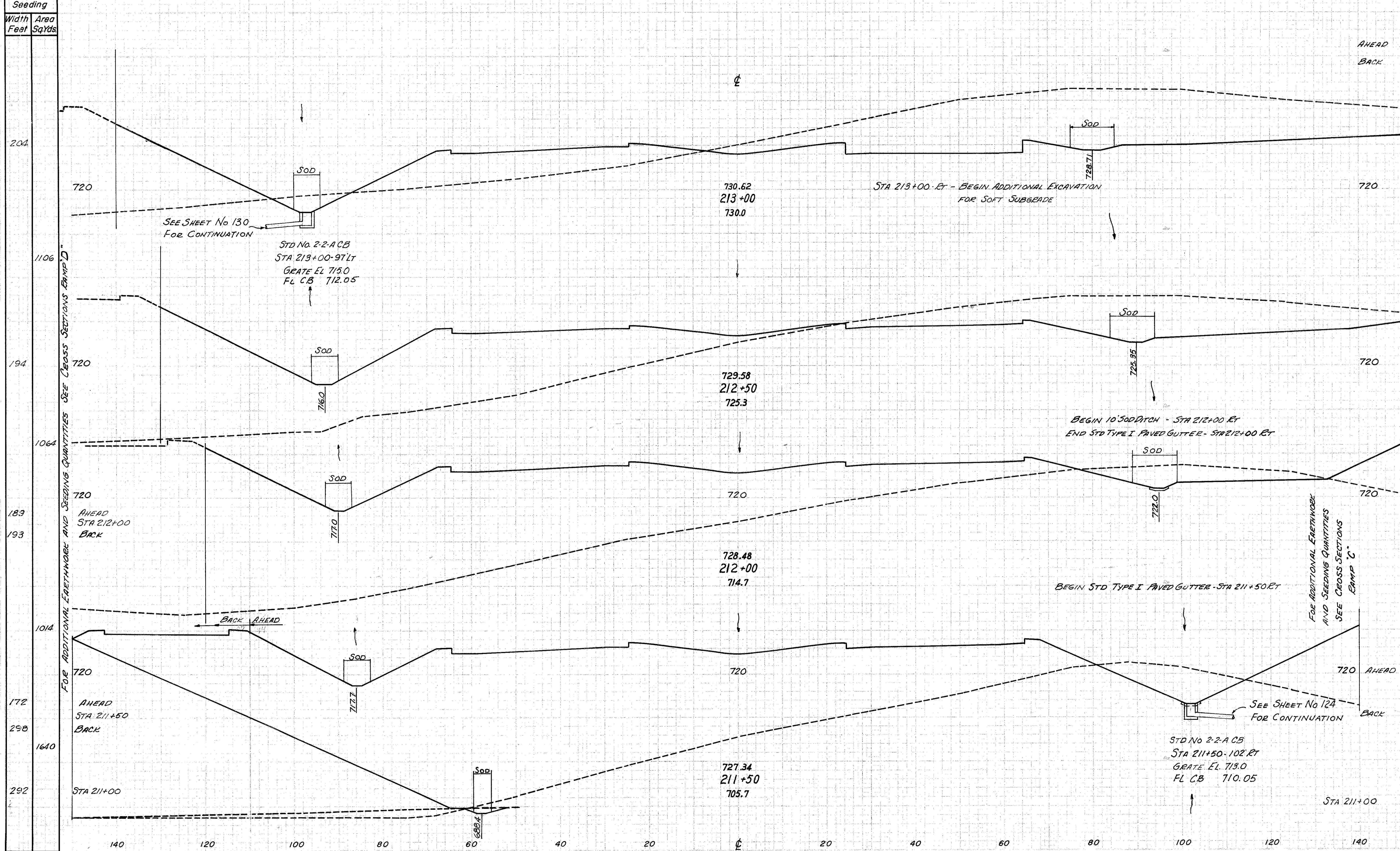
STA. 211+50 TO STA. 213+00
