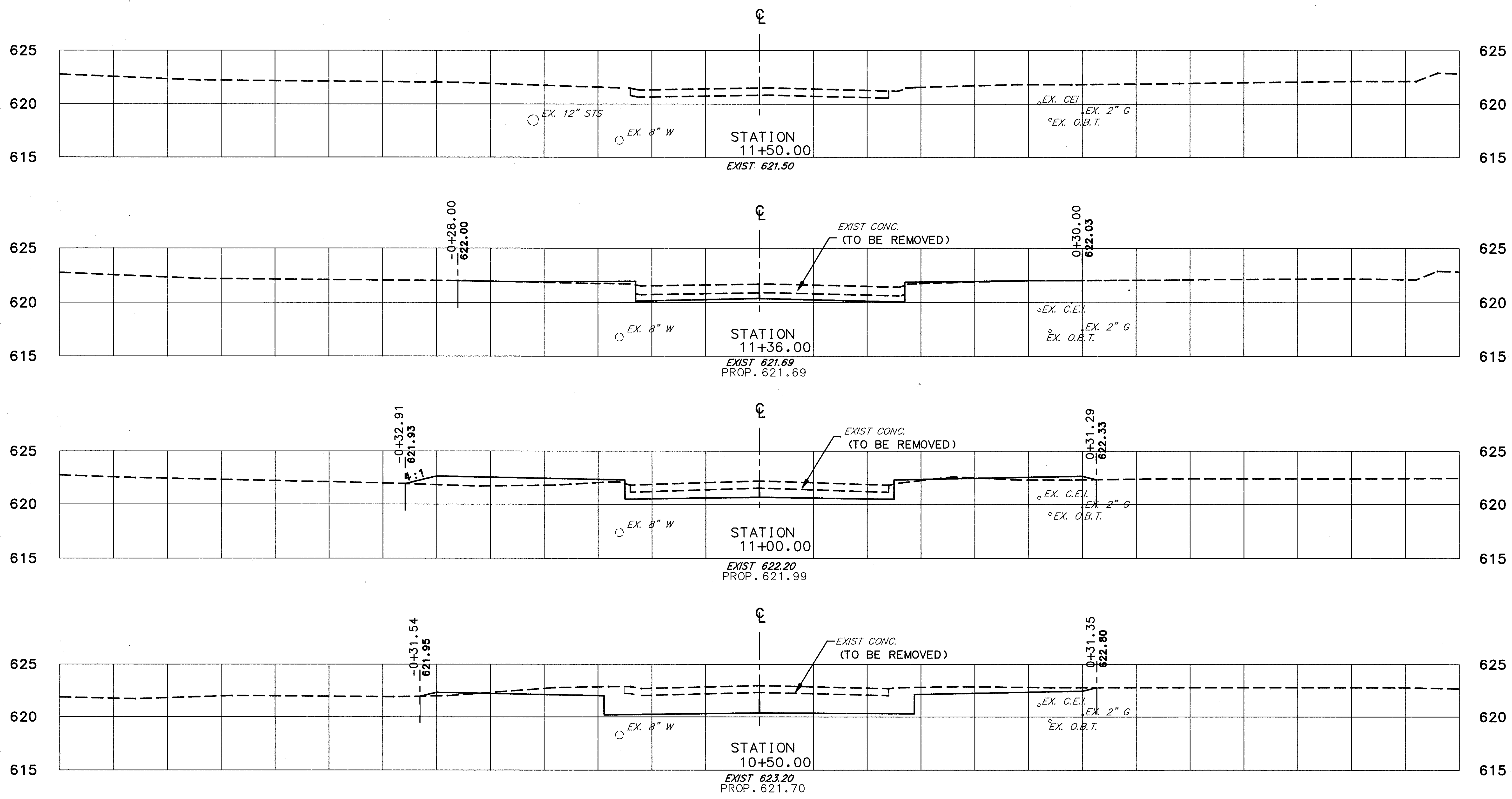
CROSS SECTIONS STA. 10+50 TO STA. 11+50
