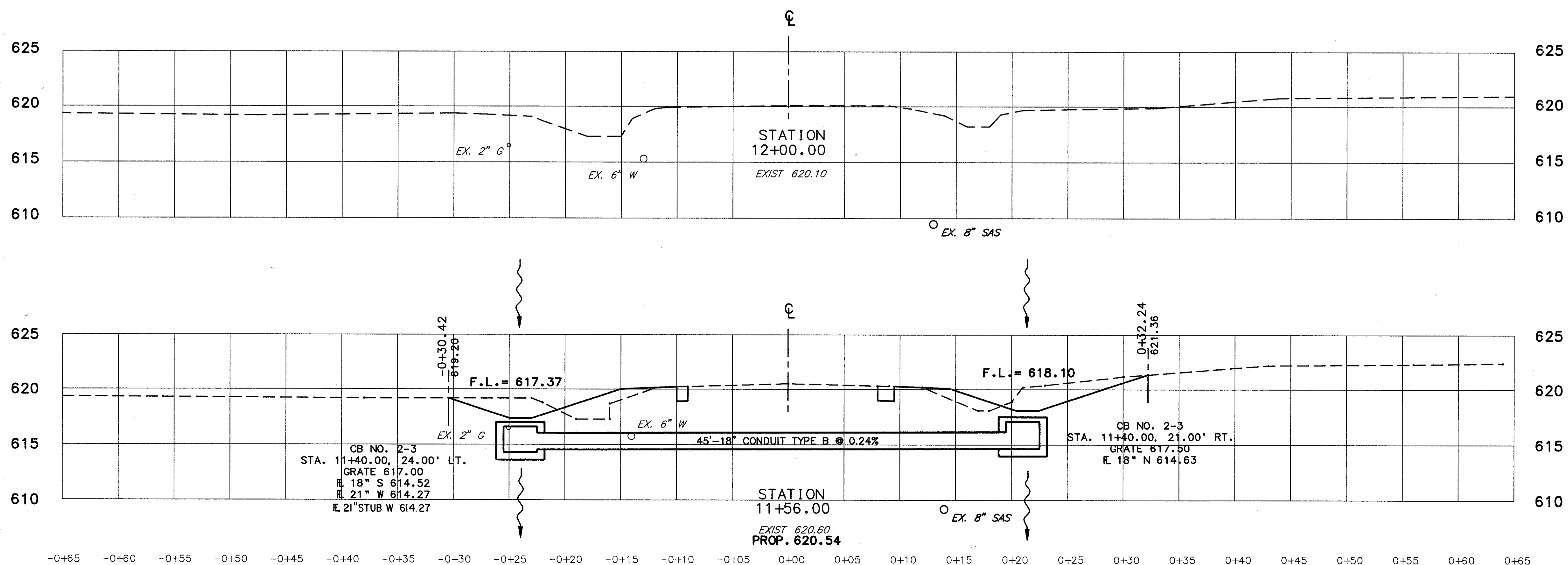
CROSS SECTIONS STA. 11+56 TO STA. 12+00
