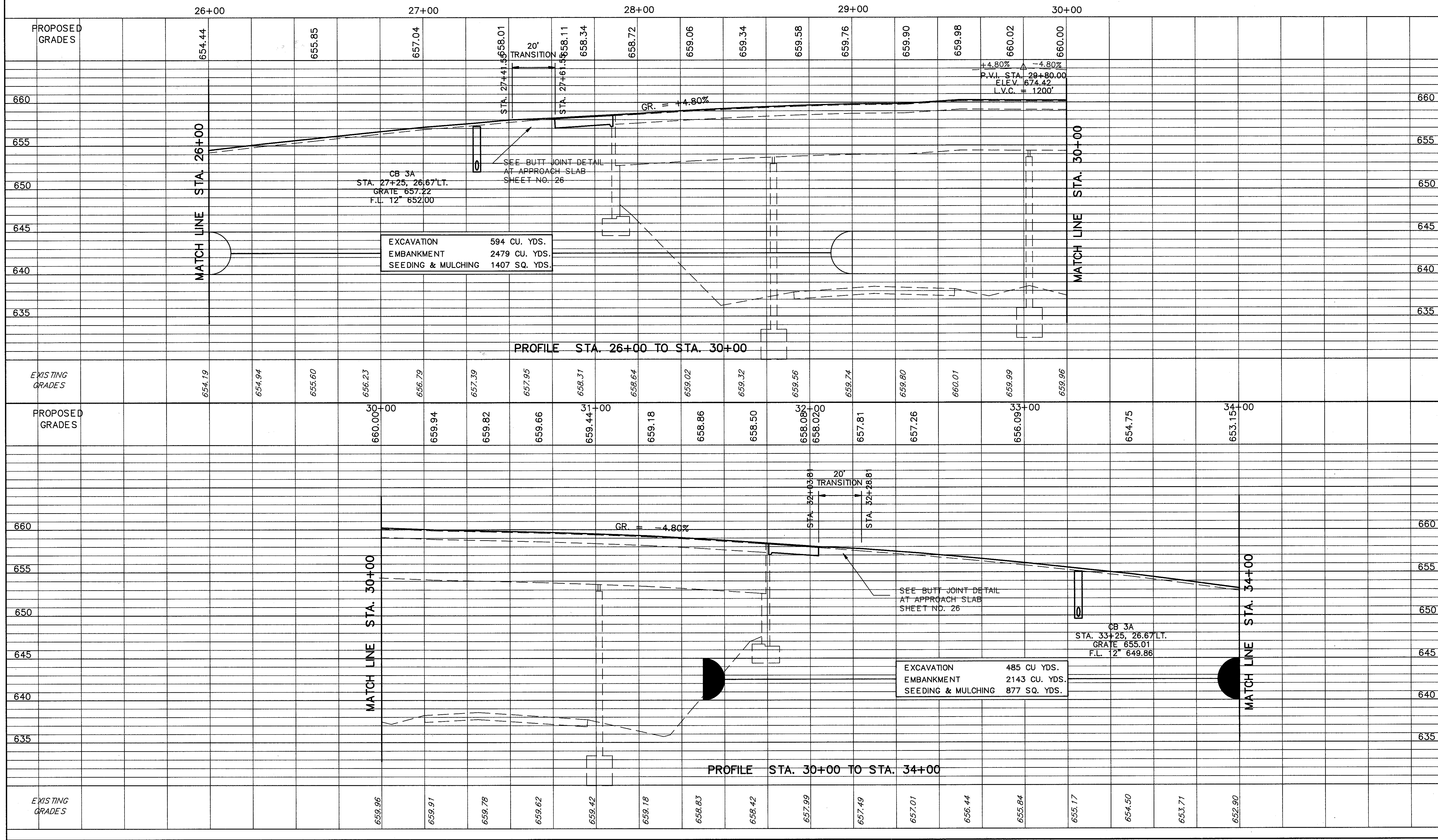
PROFILE STA. 26 + 00 TO STA. 34 + 00
