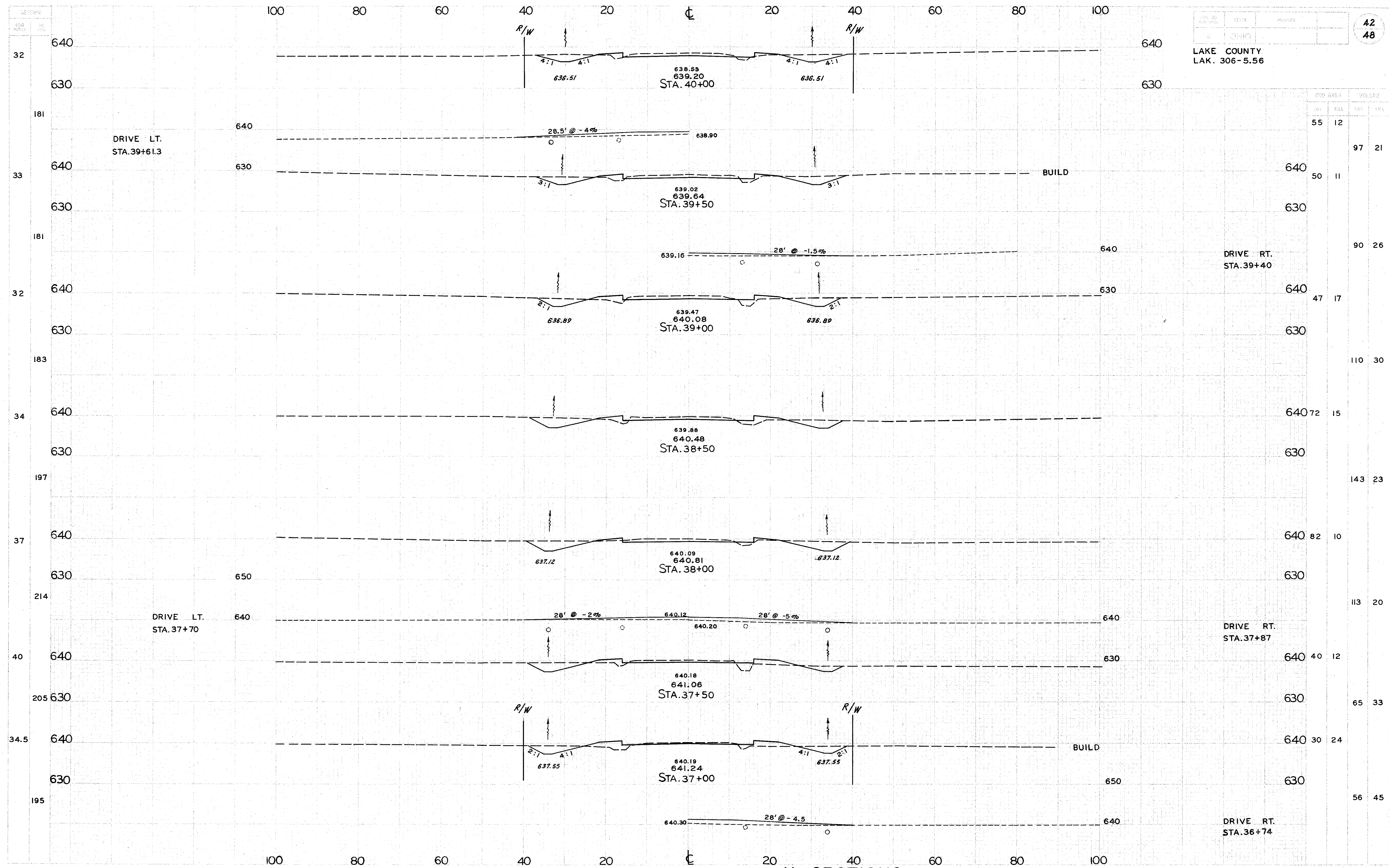
X SECTIONS S.R. 306 STA. 37+00 TO STA. 40+00
