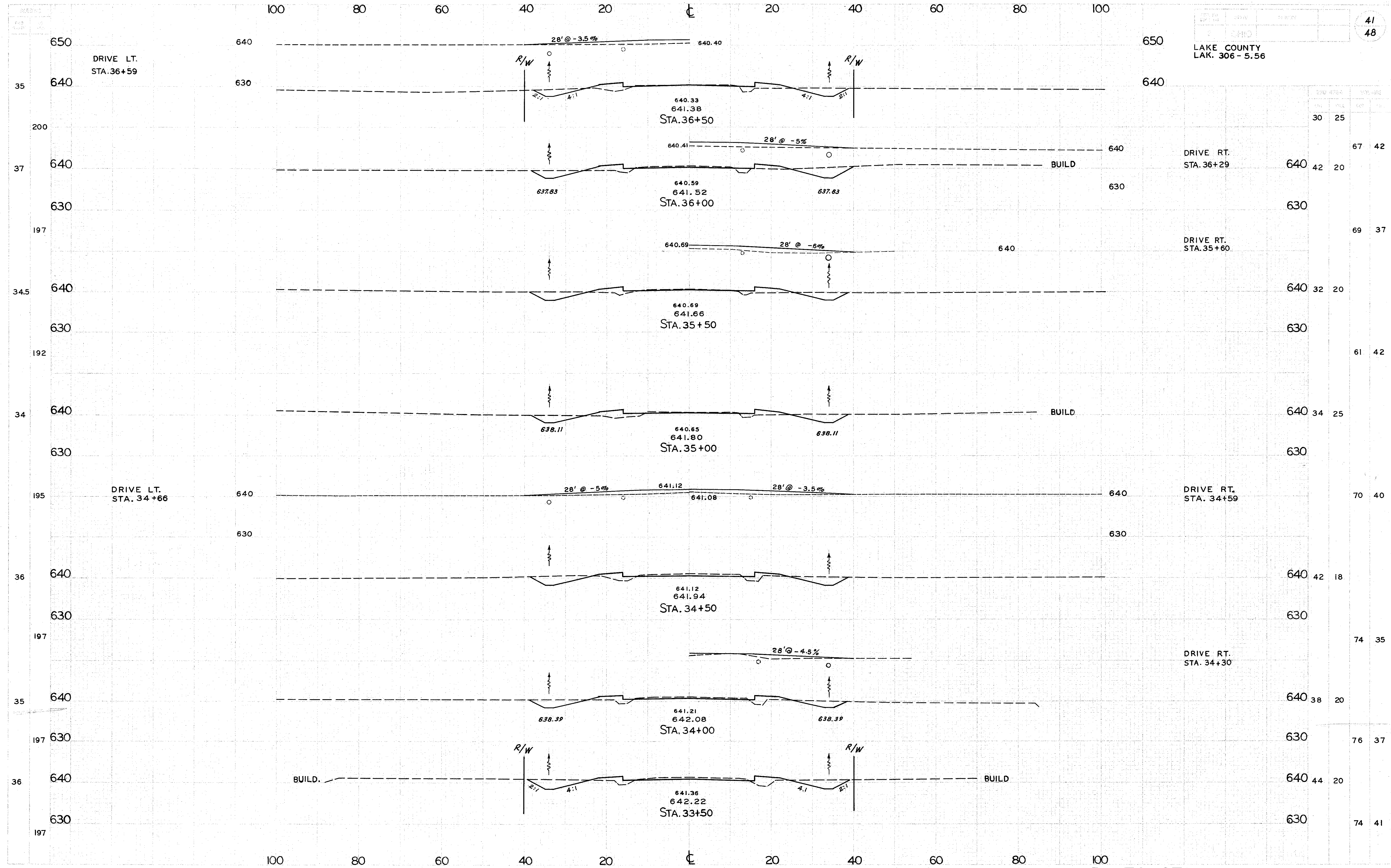
X SECTIONS S.R. 306 STA. 33+50 TO STA. 36+50
