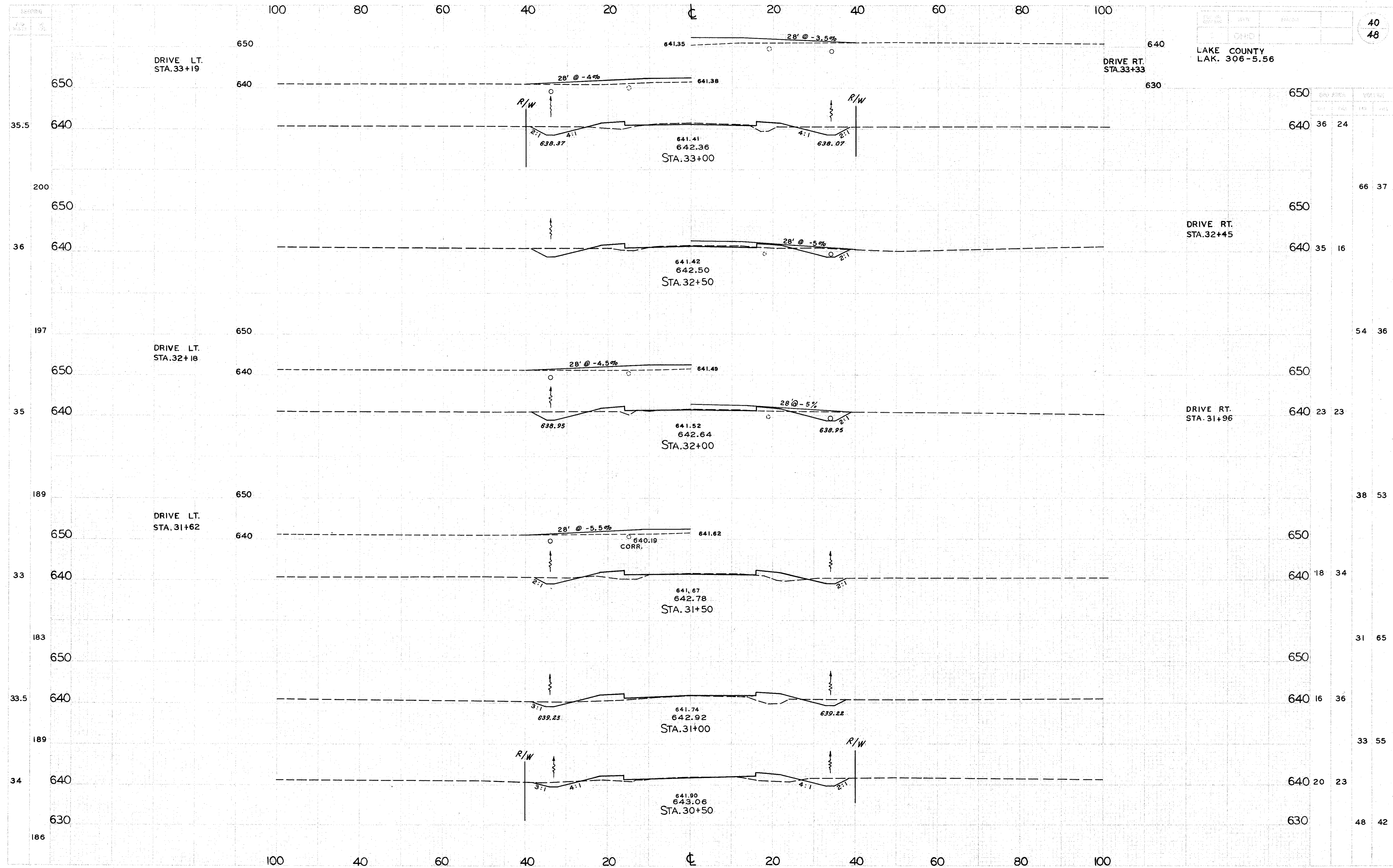
X SECTIONS S.R. 306 STA. 30+50 TO STA. 33+00
