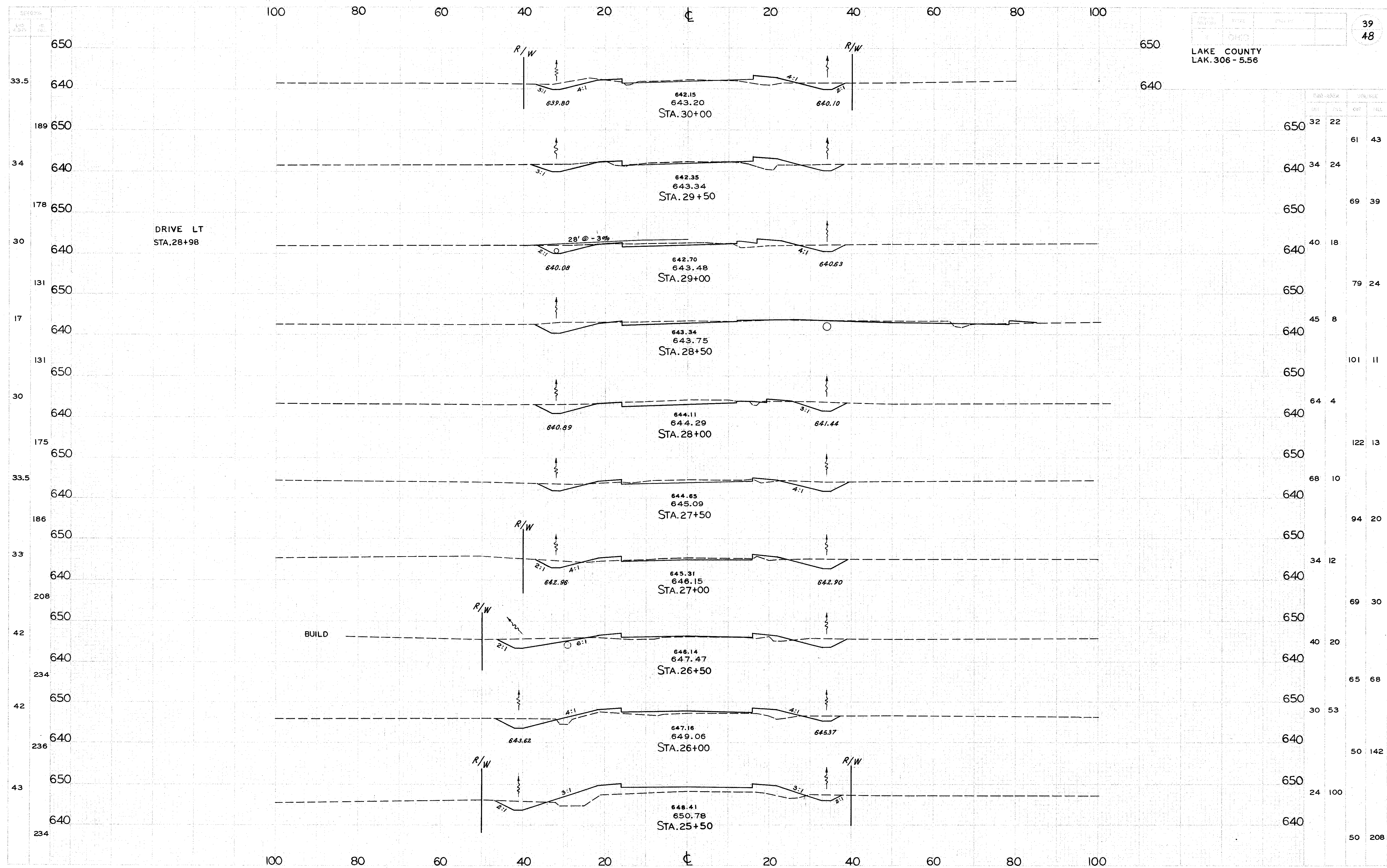
X SECTIONS S. R. 306 STA. 25+50 TO STA. 30+00
