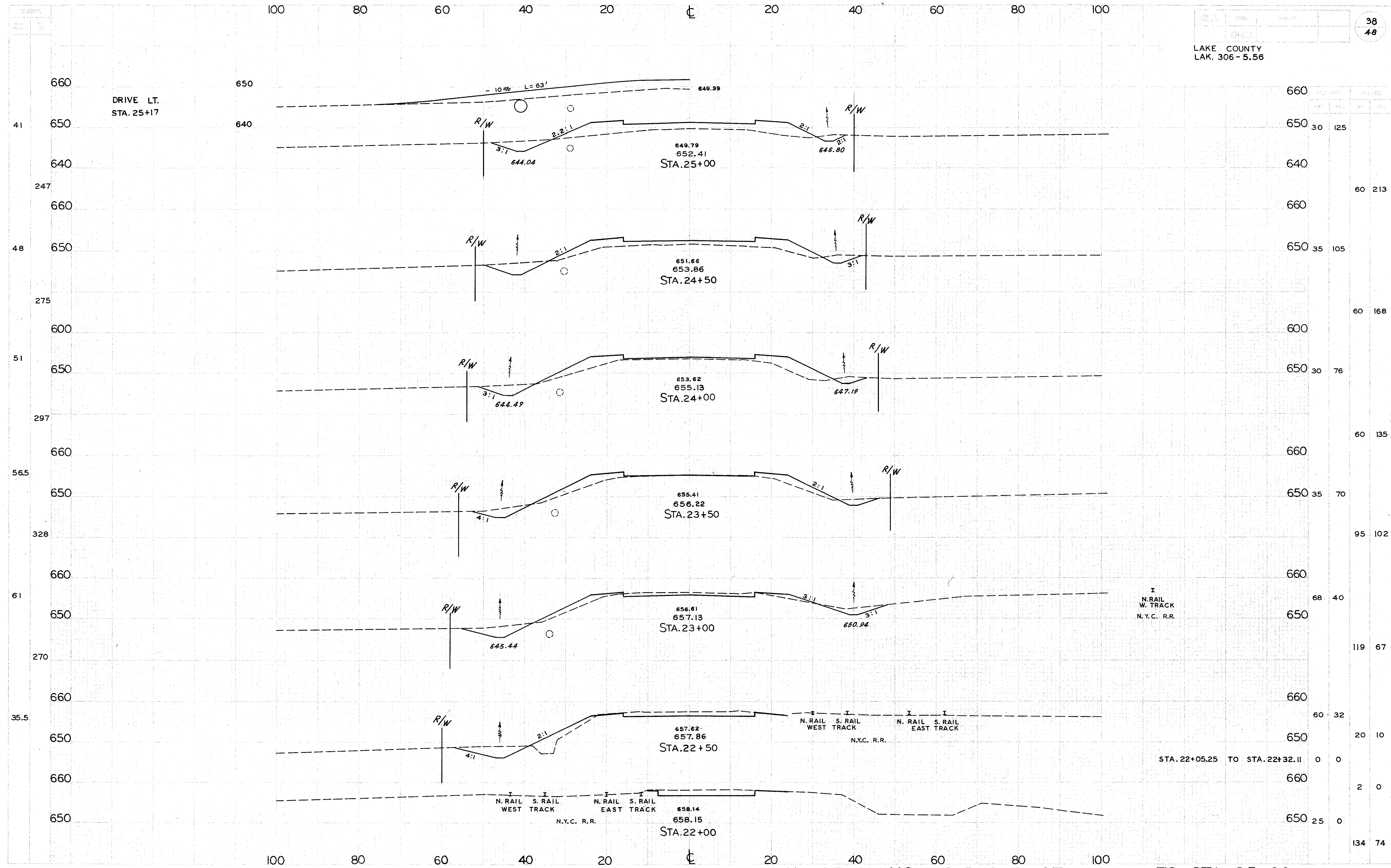
X - SECTIONS S. R. 306 STA. 22+00 TO STA. 25+00
