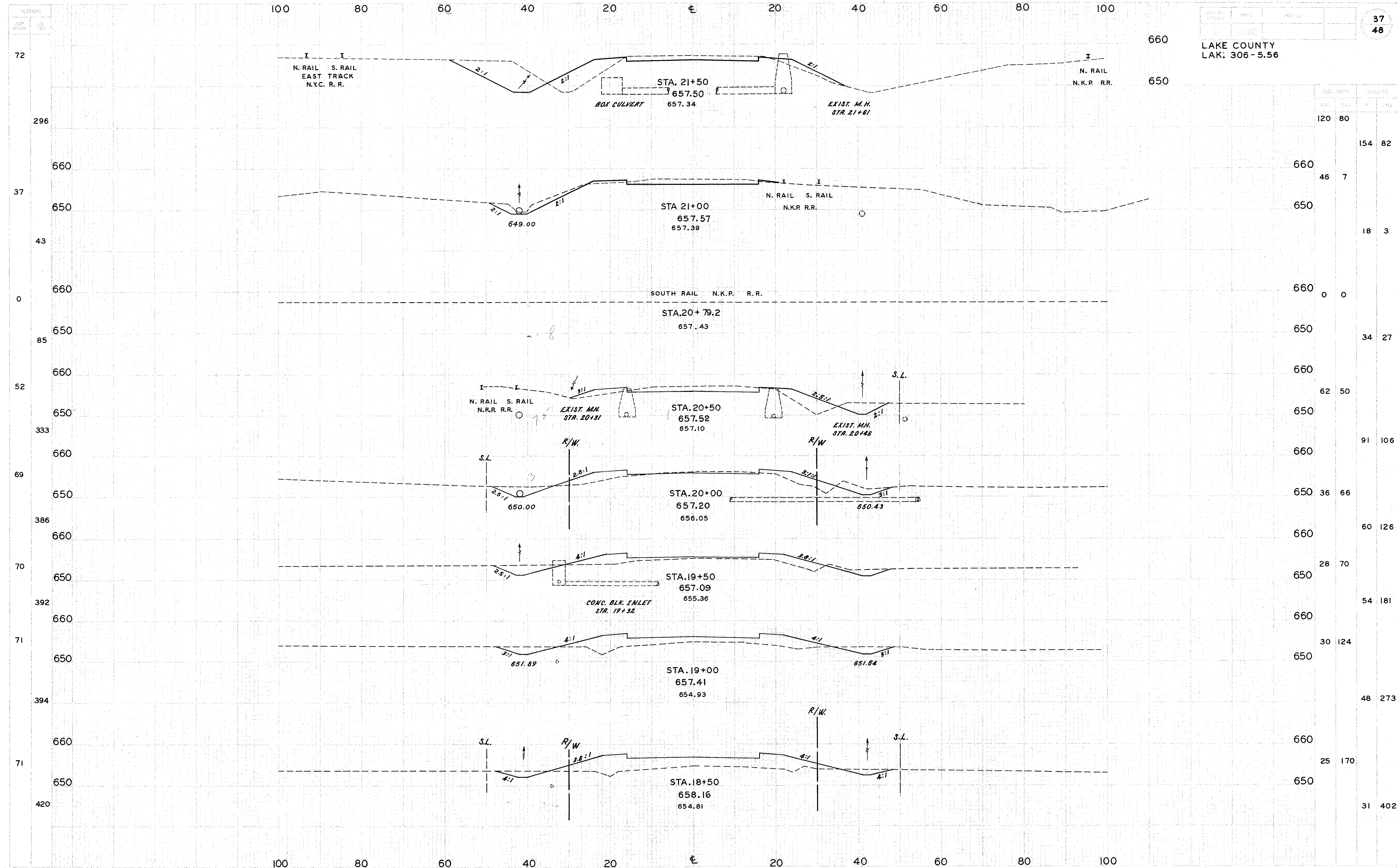
X-SECTIONS S.R. 306 STA. 18+50 TO STA. 21+50
