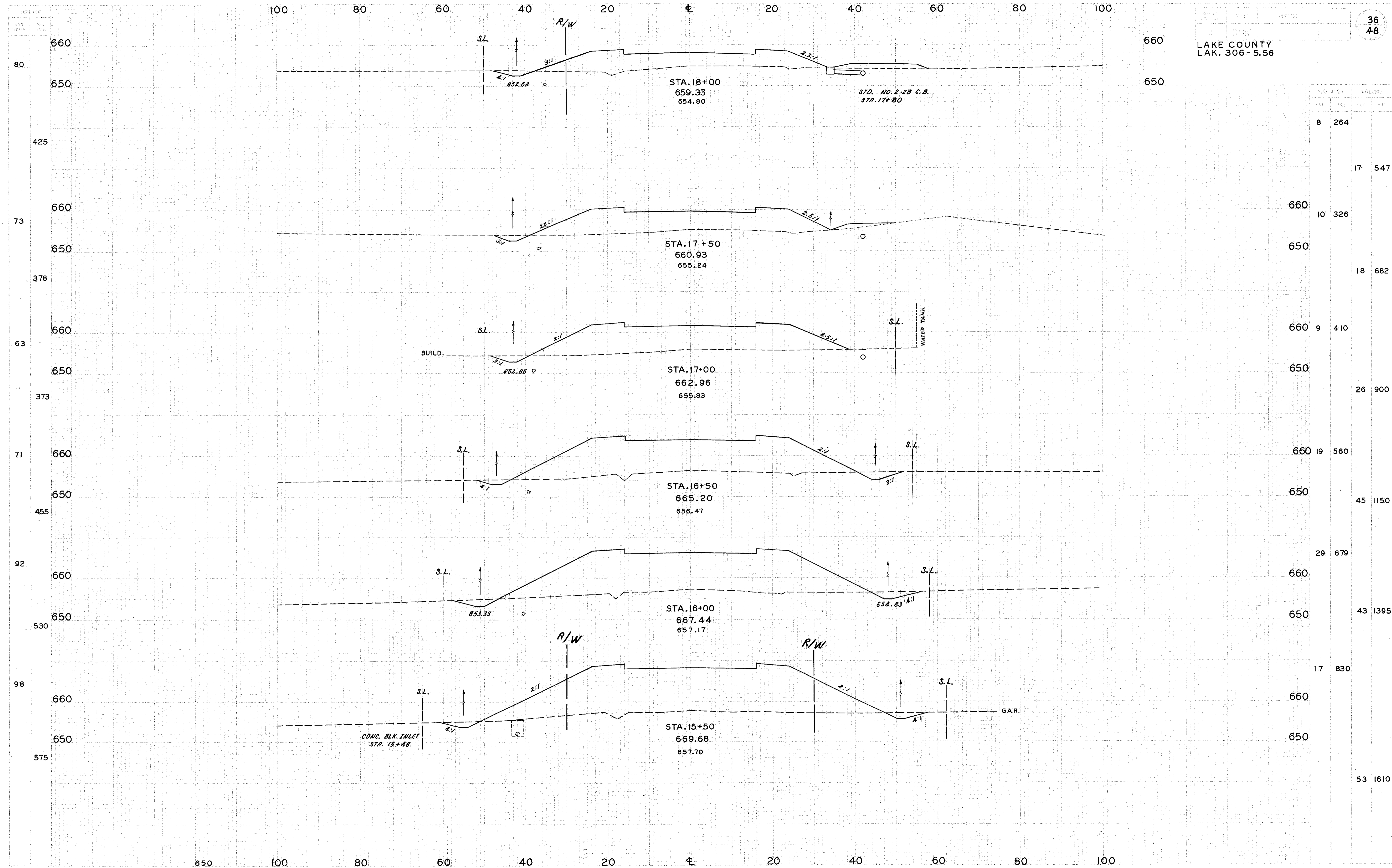
X- SECTIONS S. R. 306 STA. 15+50 TO STA. 18+00
