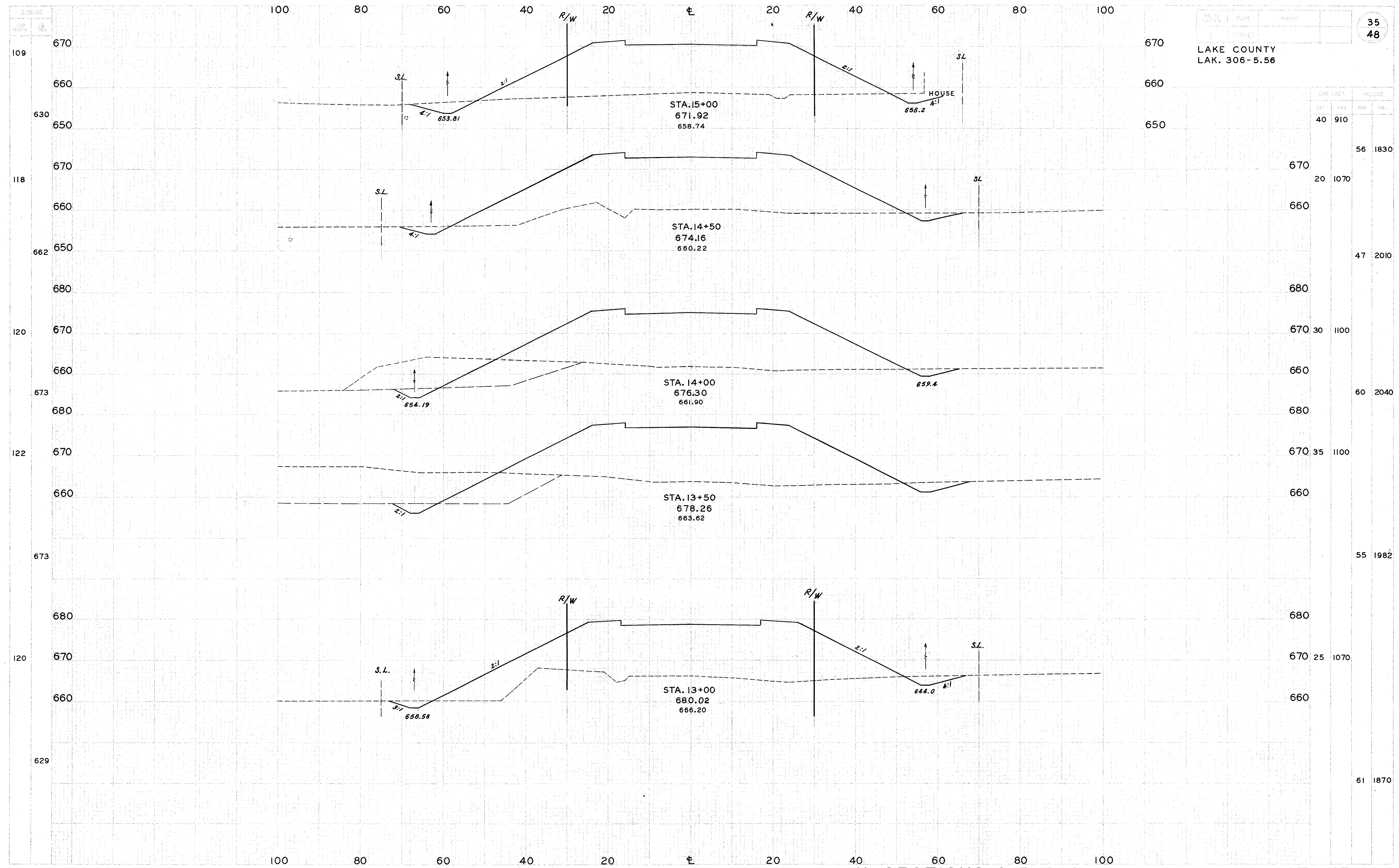
X-SECTIONS S.R. 306 STA. 13+00 TO STA. 15+00
