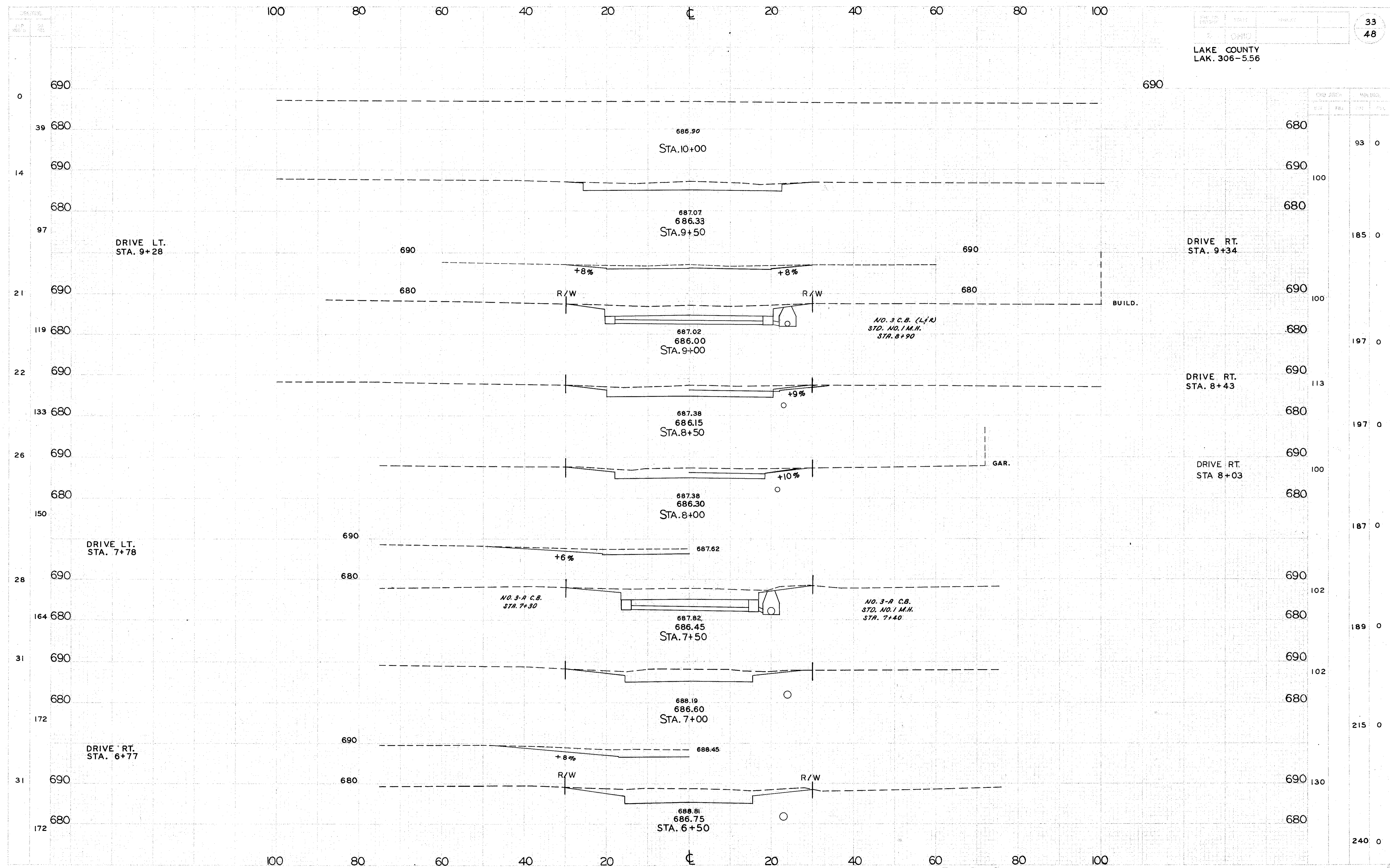
X SECTIONS S.R. 306 STA. 6+50 TO STA. 10+00
