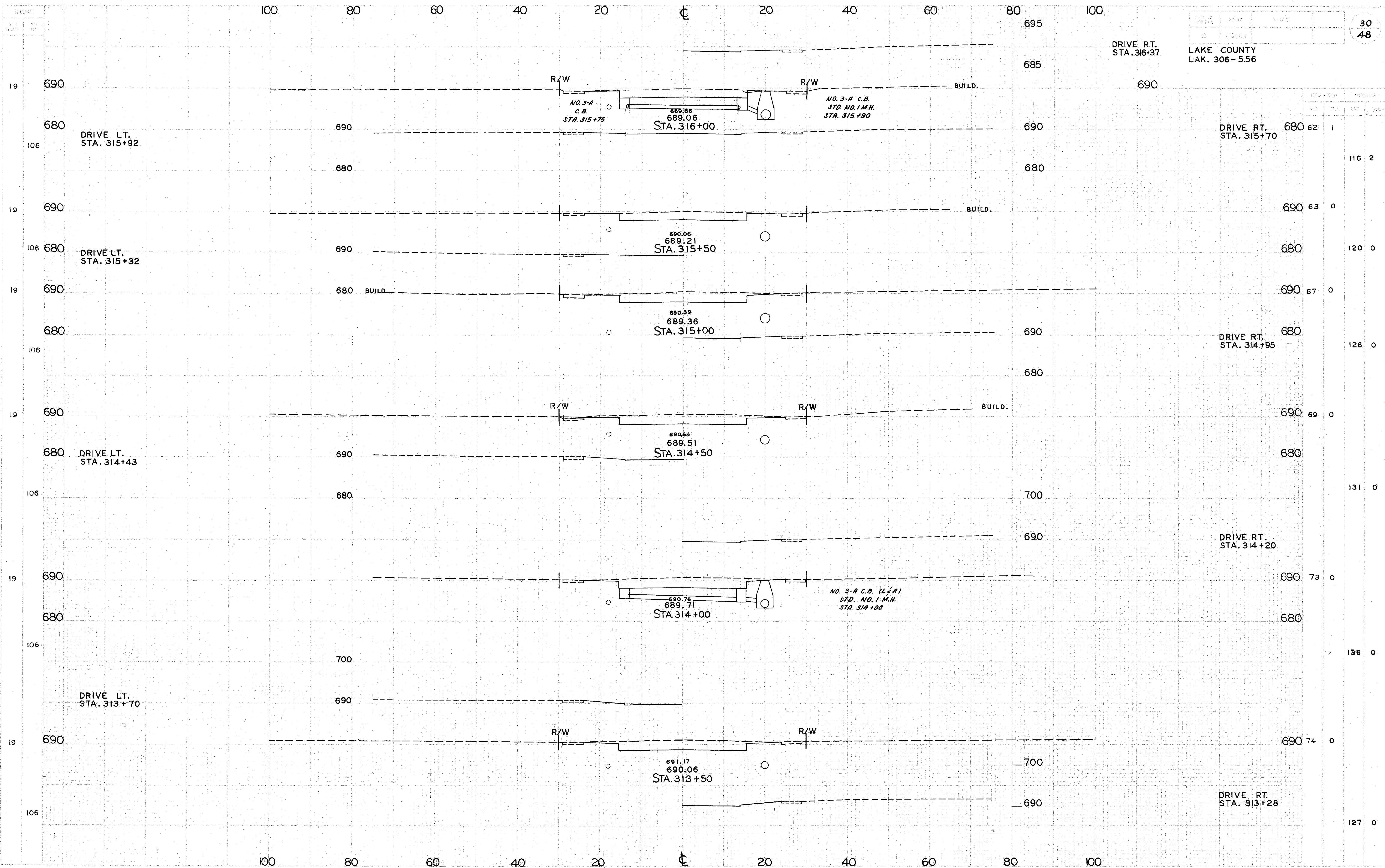
X SECTIONS S.R. 306 STA. 313+50 TO STA. 316+00
