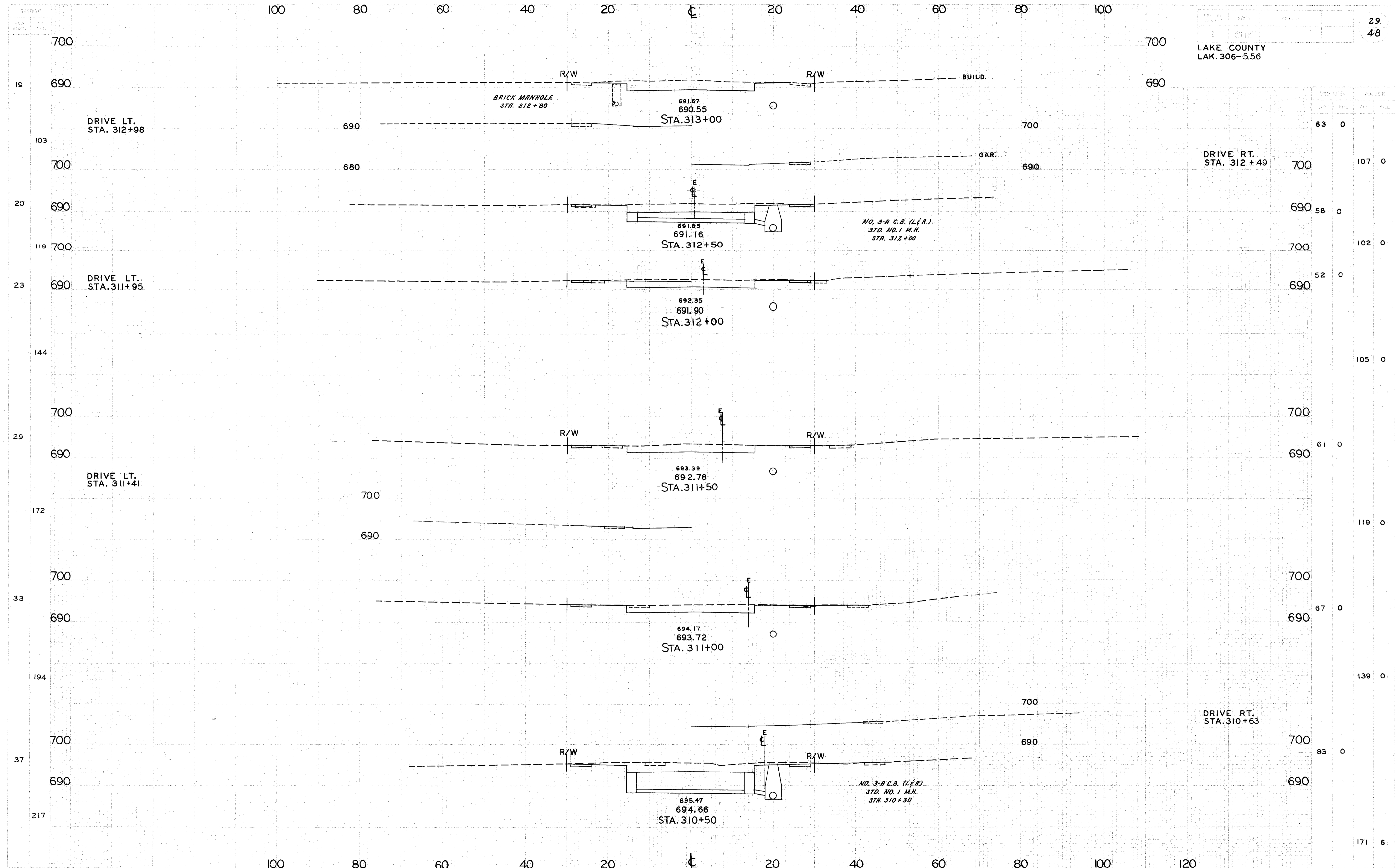
X SECTIONS S. R. 306 STA. 310+50 TO STA. 313+00
