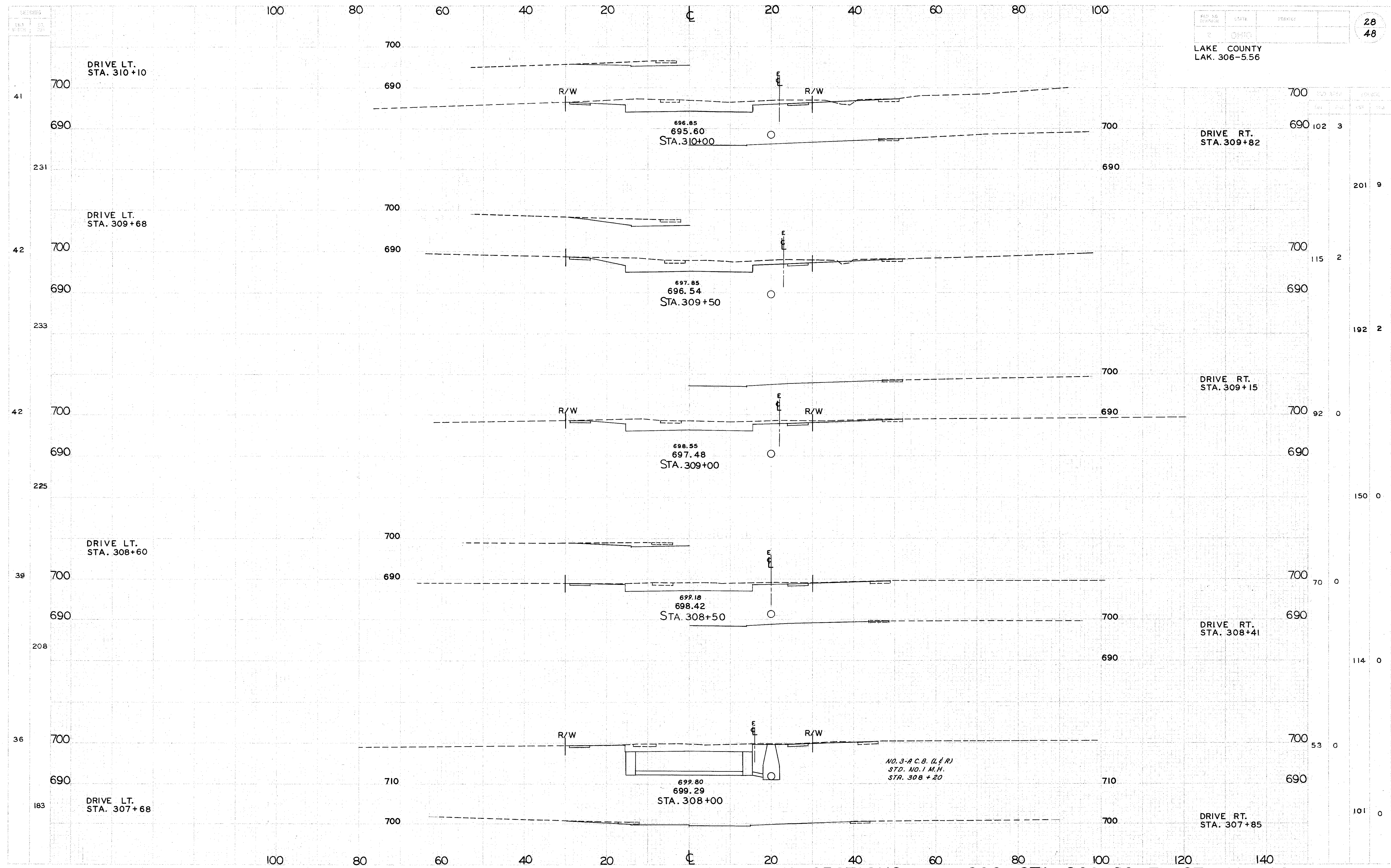
X SECTIONS S. R. 306 STA. 308+00 TO STA. 310+00
