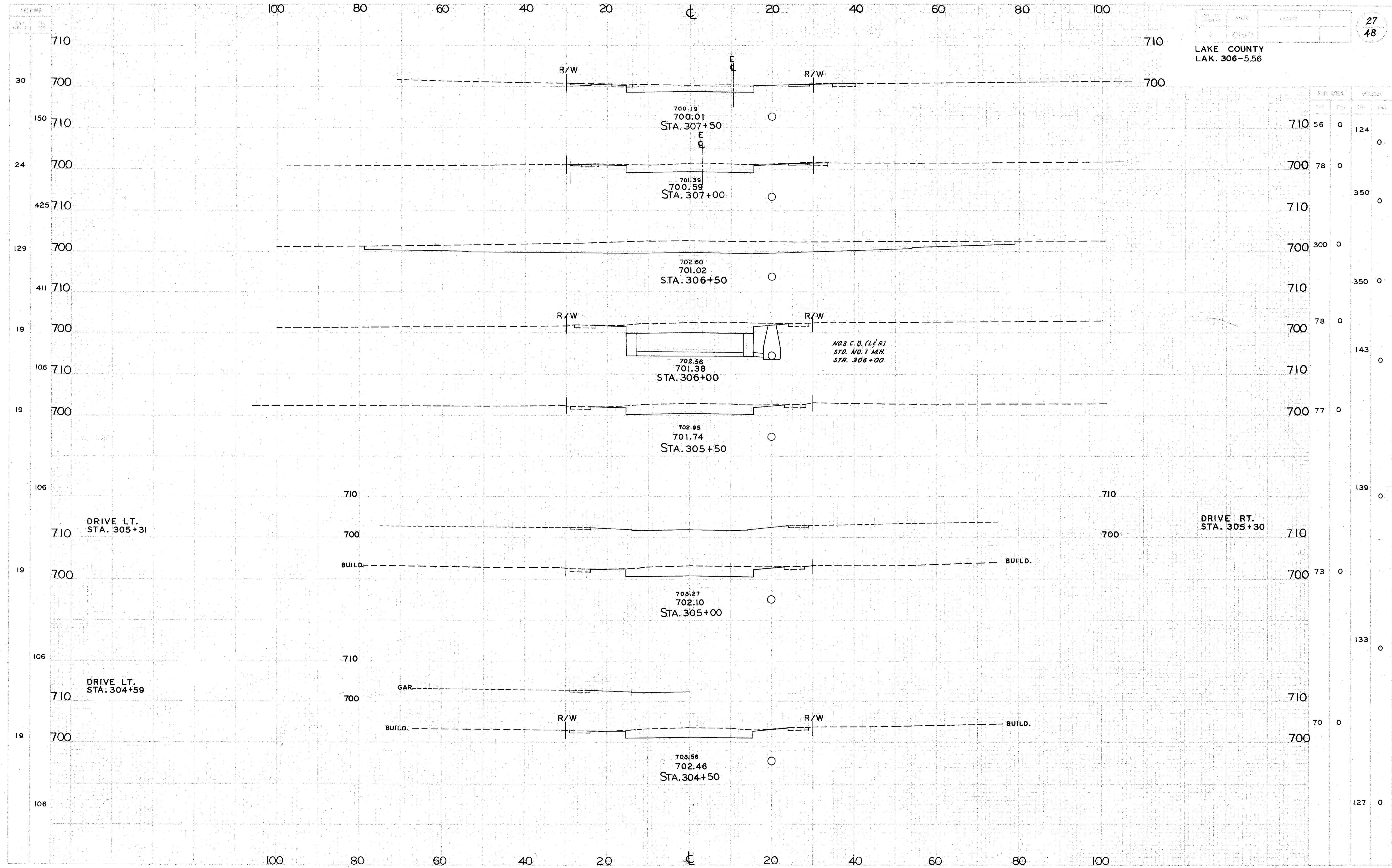
X SECTIONS S. R. 306 STA. 304+50 TO STA. 307+50
