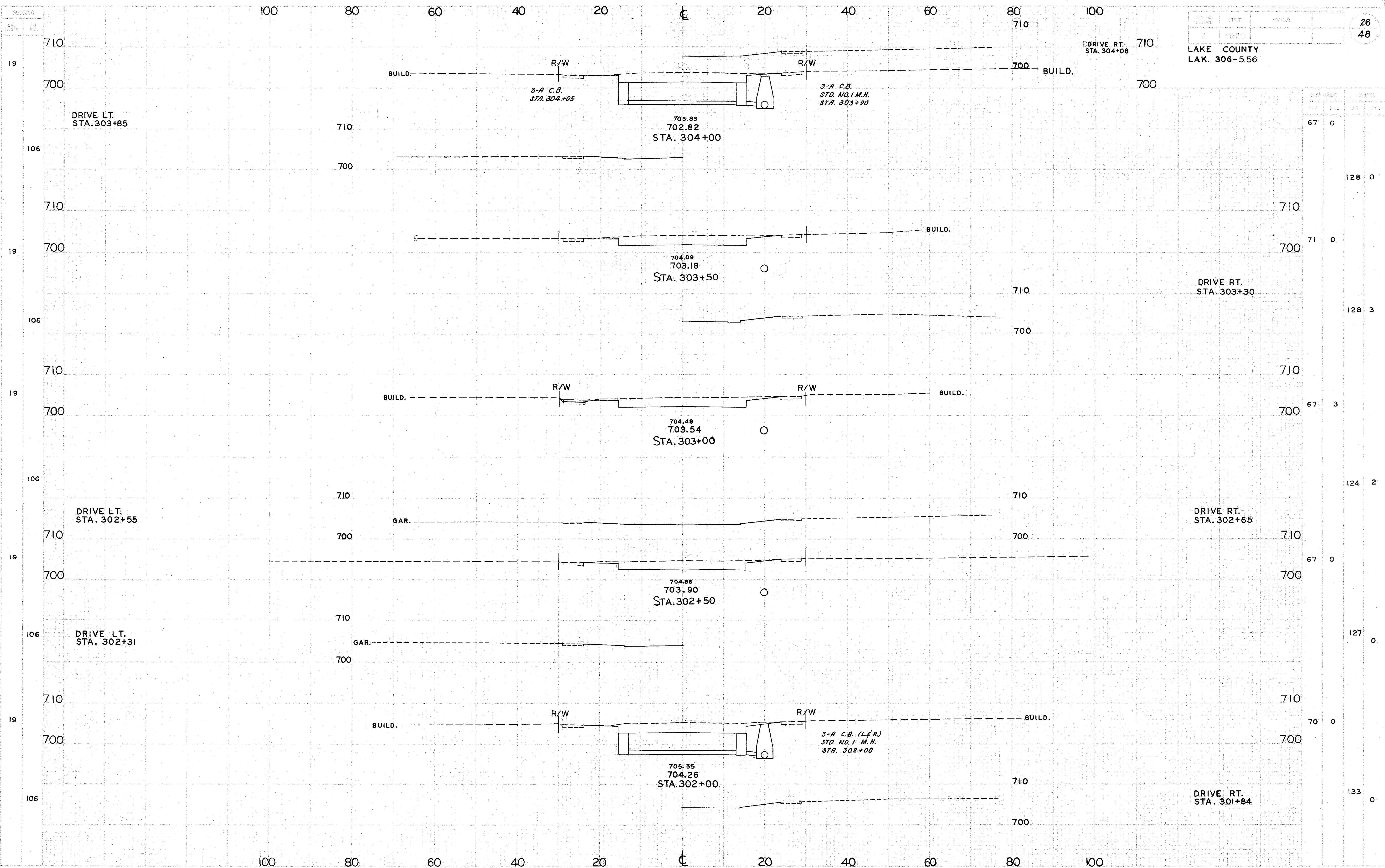
X SECTIONS S. R. 306 STA. 302+00 TO STA. 304+00
