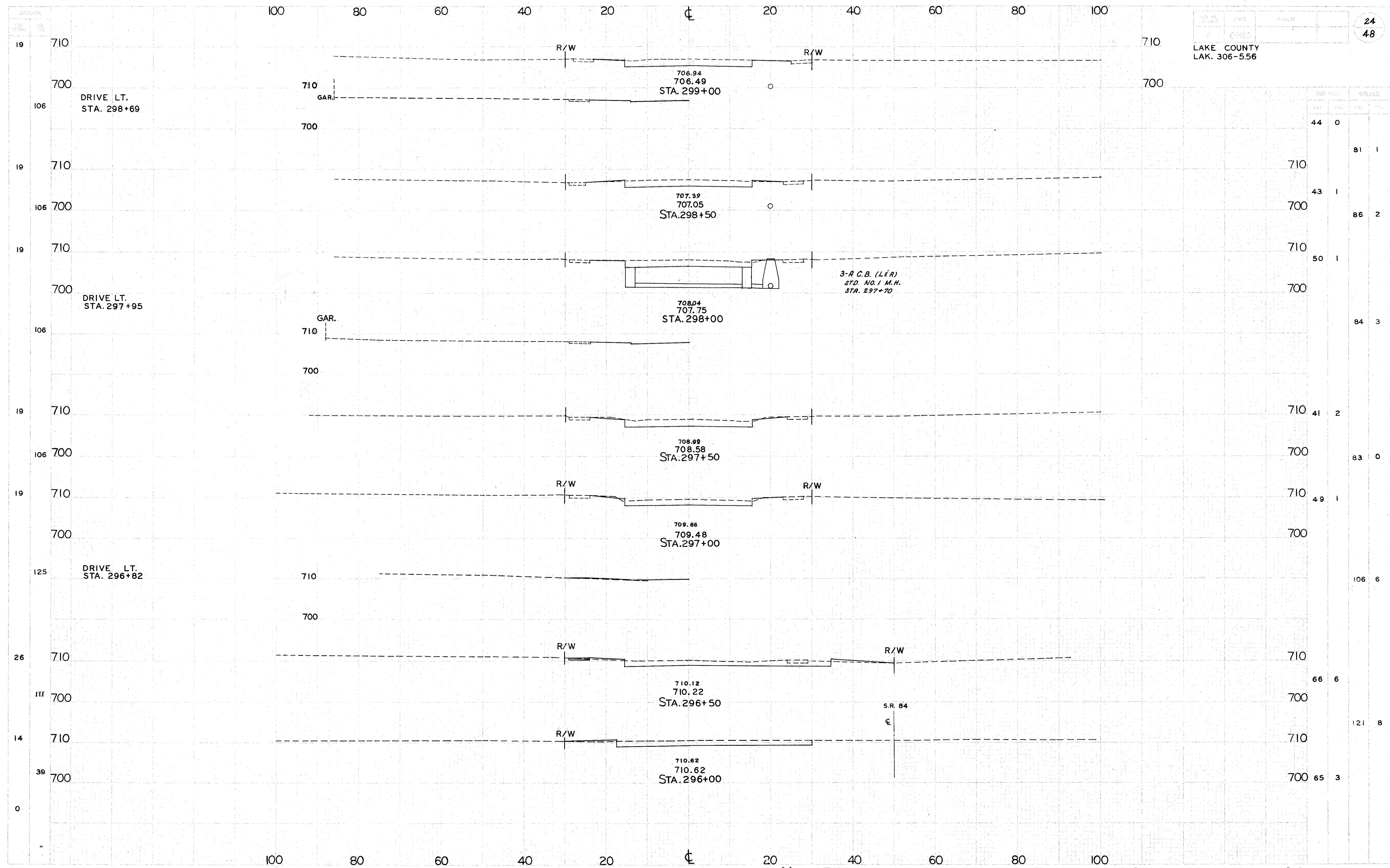
X SECTIONS S. R. 306 STA. 296+00 TO STA. 299+00
