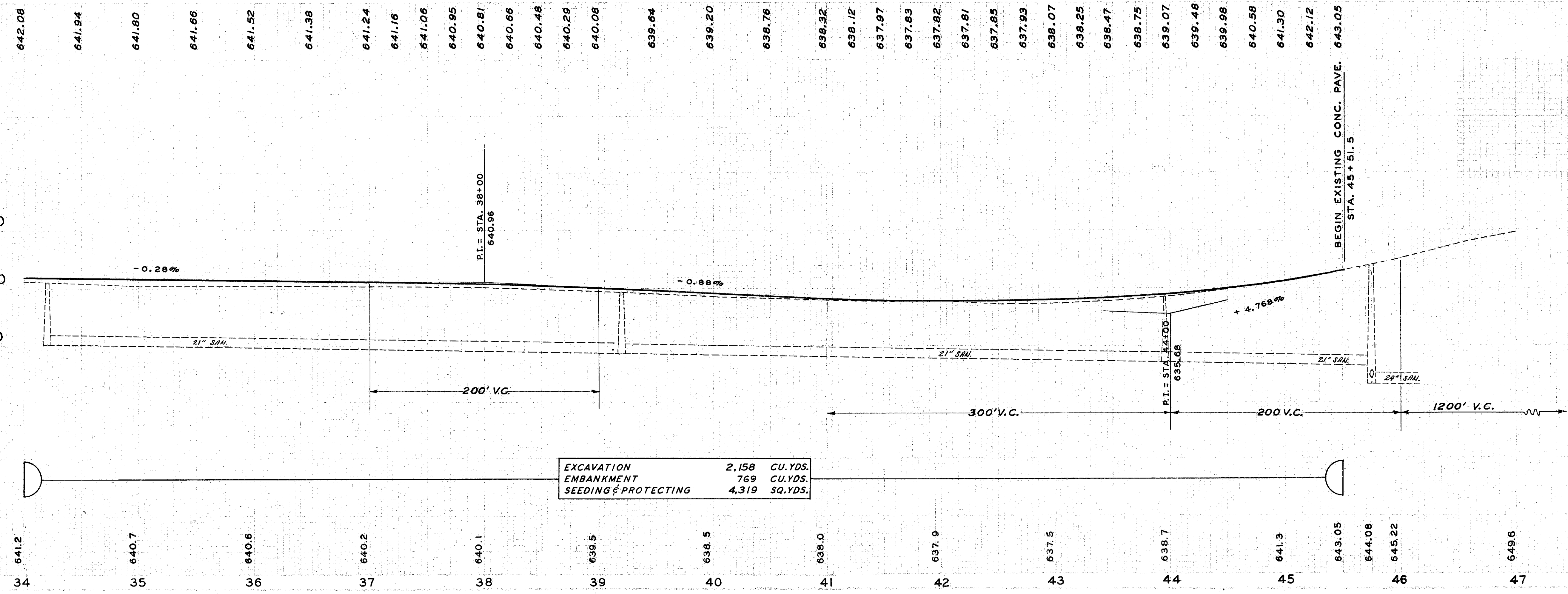
S.R. 306 PLAN & PROFILE STA. 34+00 TO STA. 46+00
