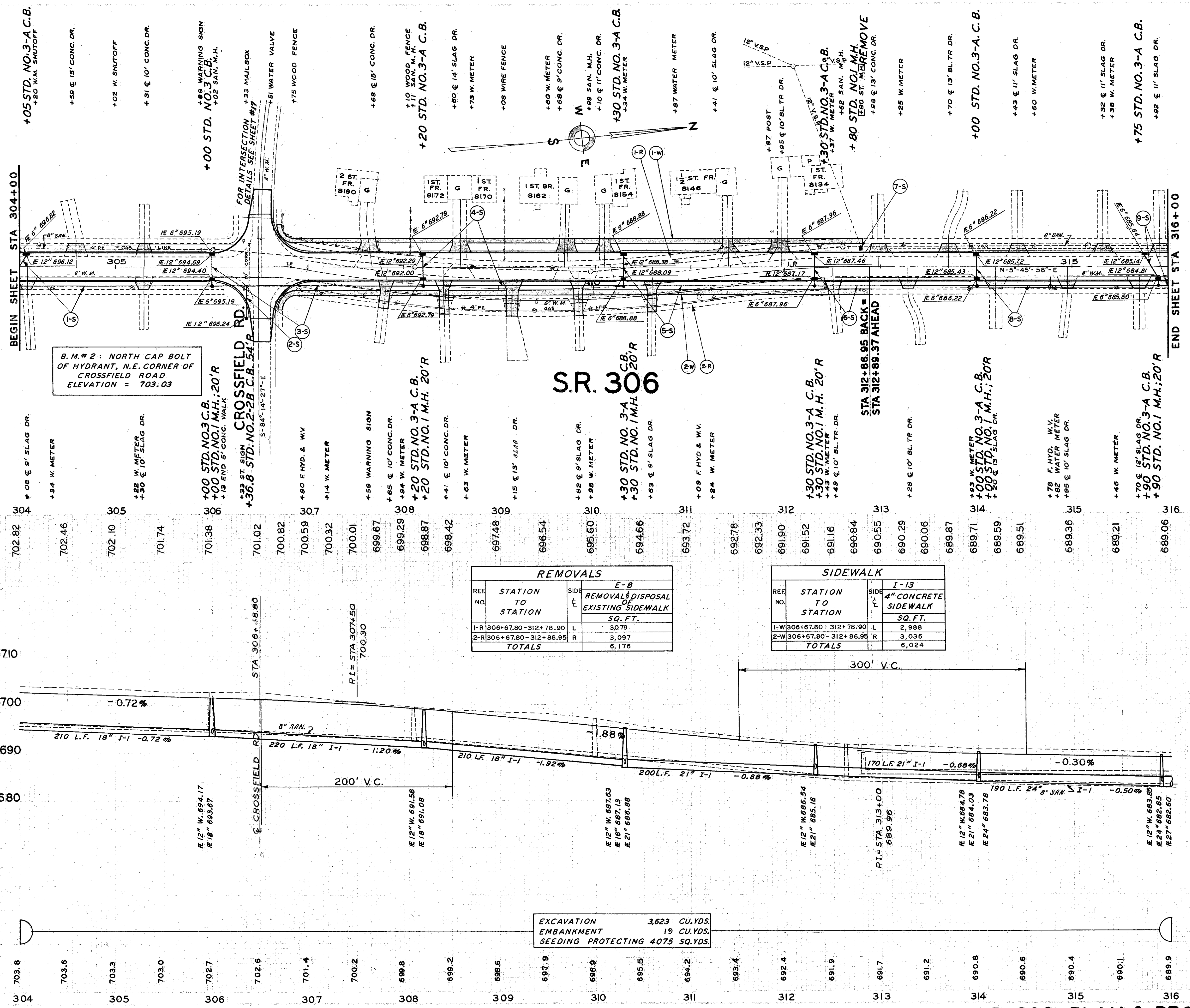
S.R. 306 PLAN & PROFILE STA 304+00 TO STA 316+00
