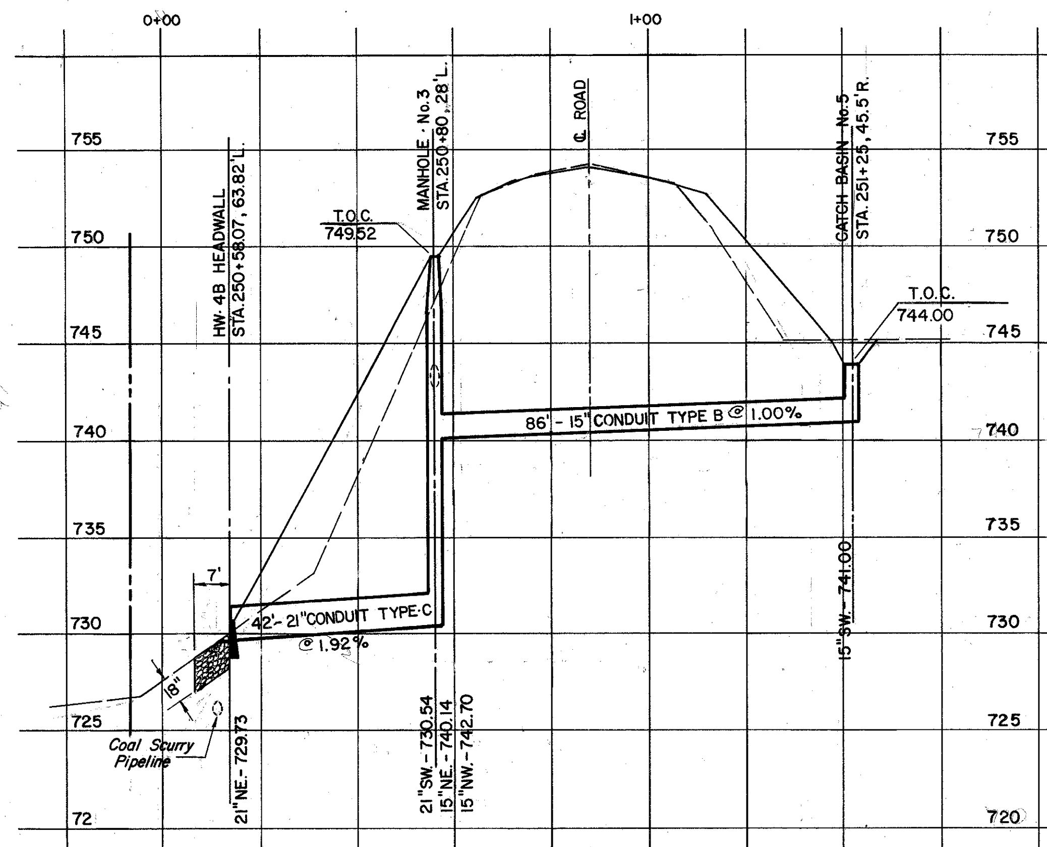
CROSS - OVER STA. 250+97.14
