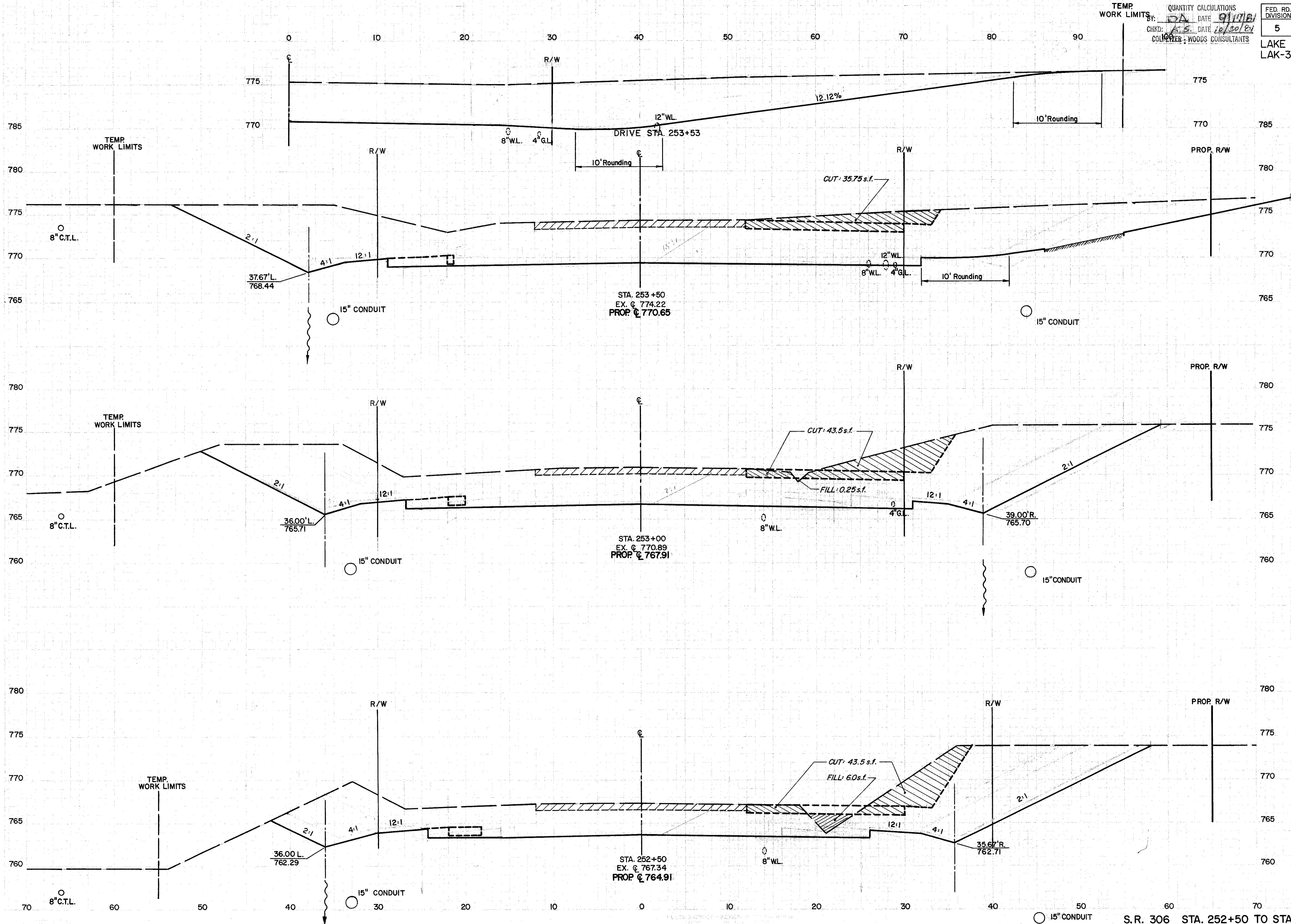
S.R. 306 STA. 252+50 TO STA. 253+50
