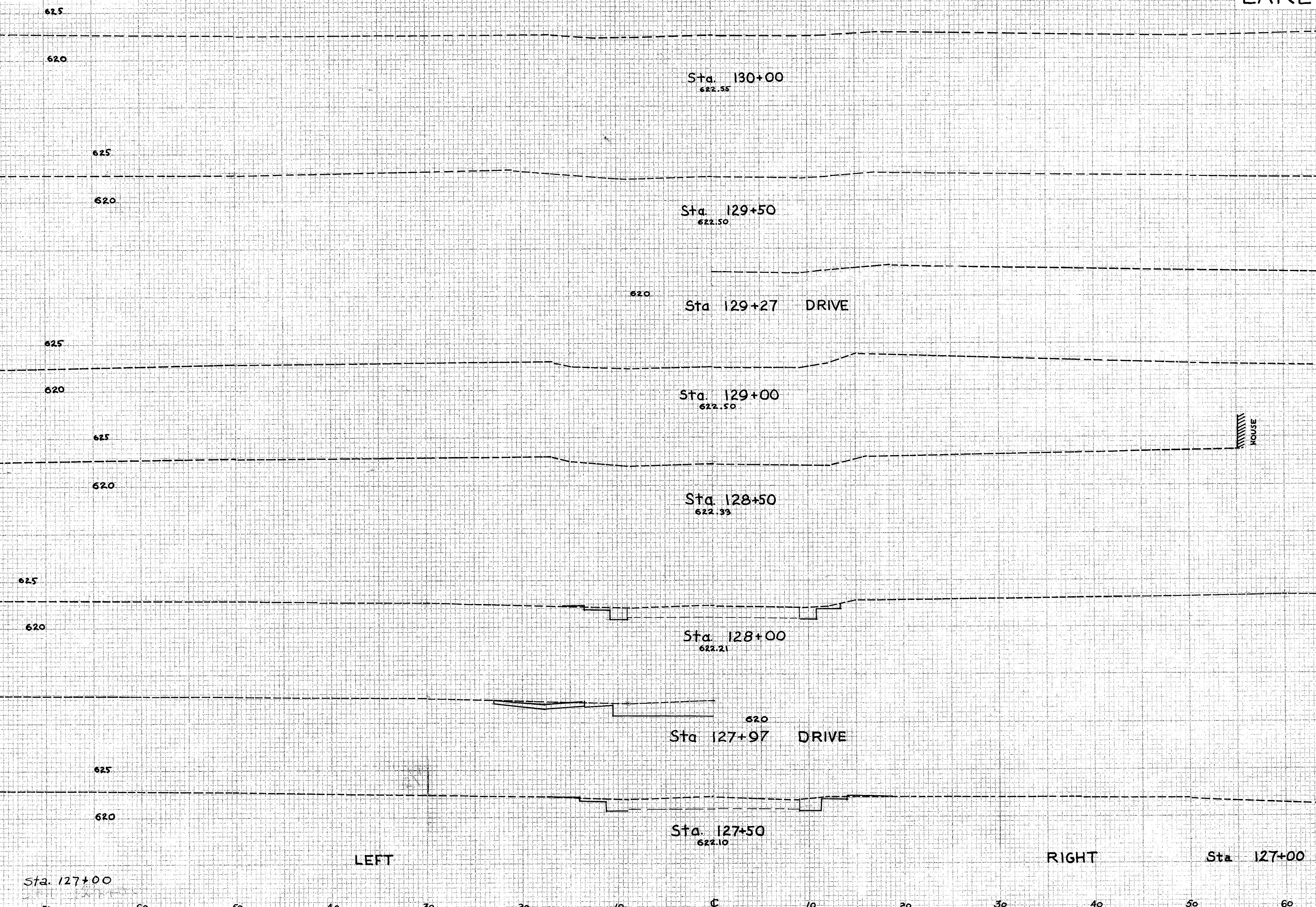
X-SECTIONS STA. 127+50 TO STA. 130+00
