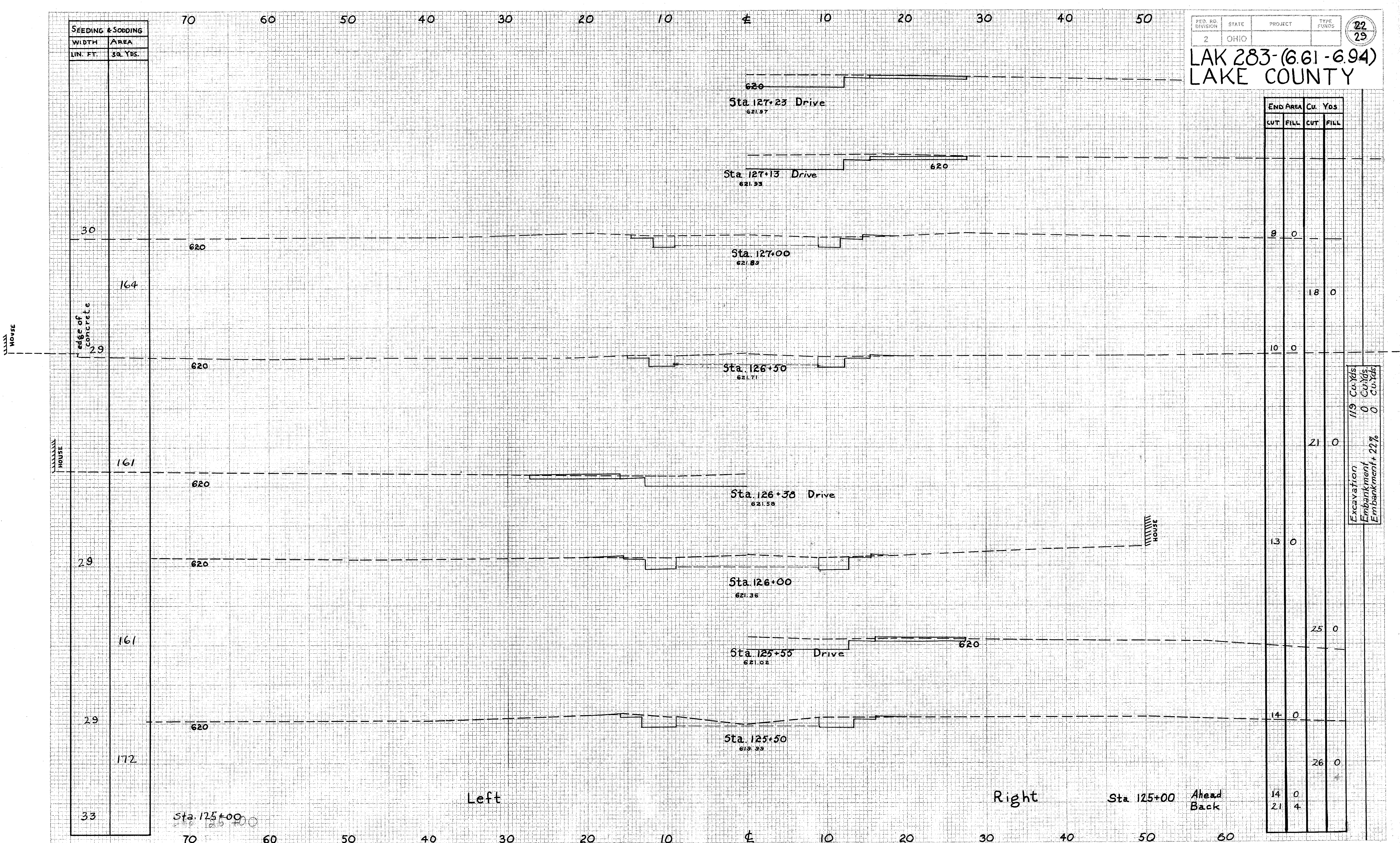
X-SECTIONS STA. 125+50 TO STA. 127+00
