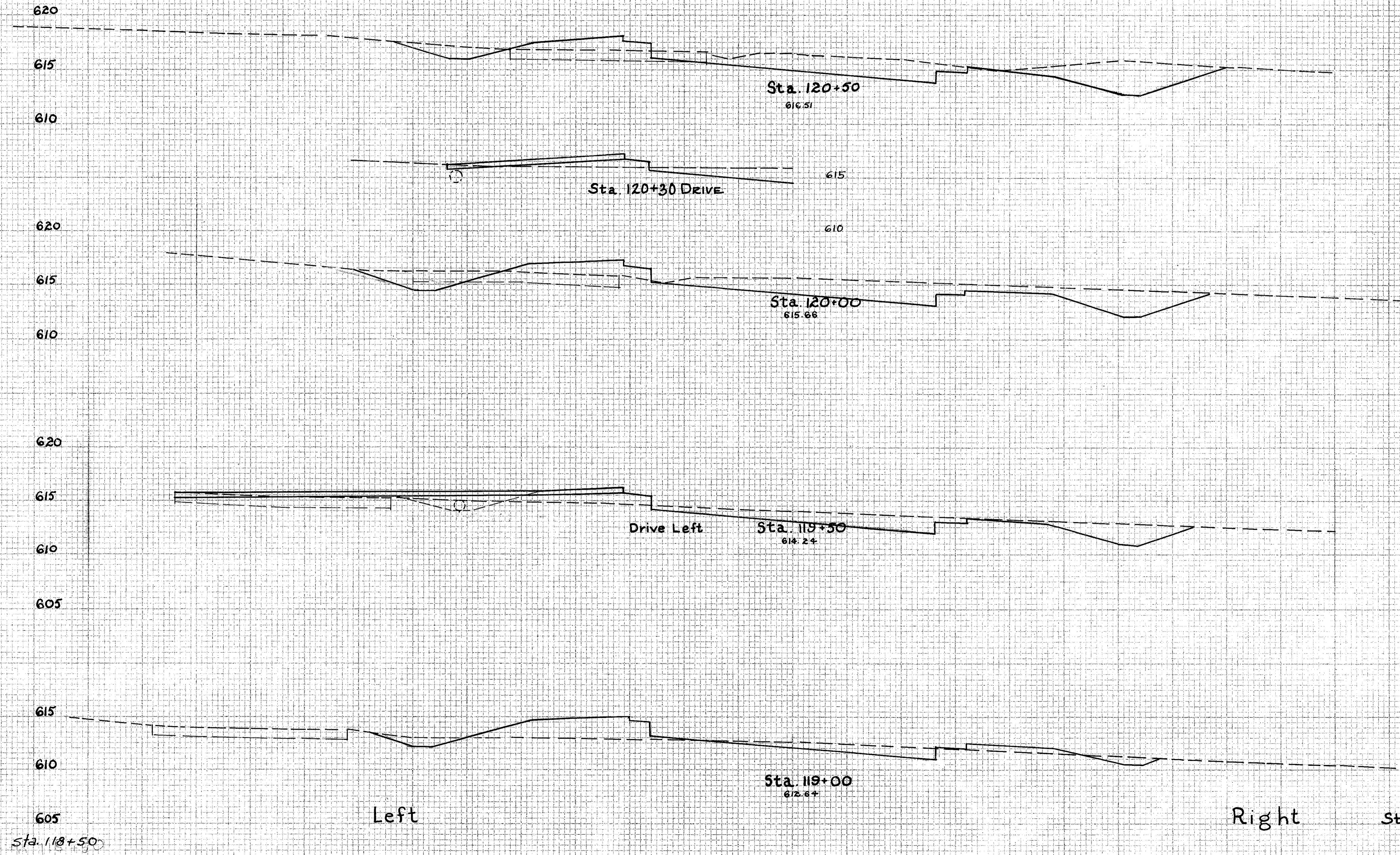
X-SECTIONS STA. 119+00 TO STA. 120+50
