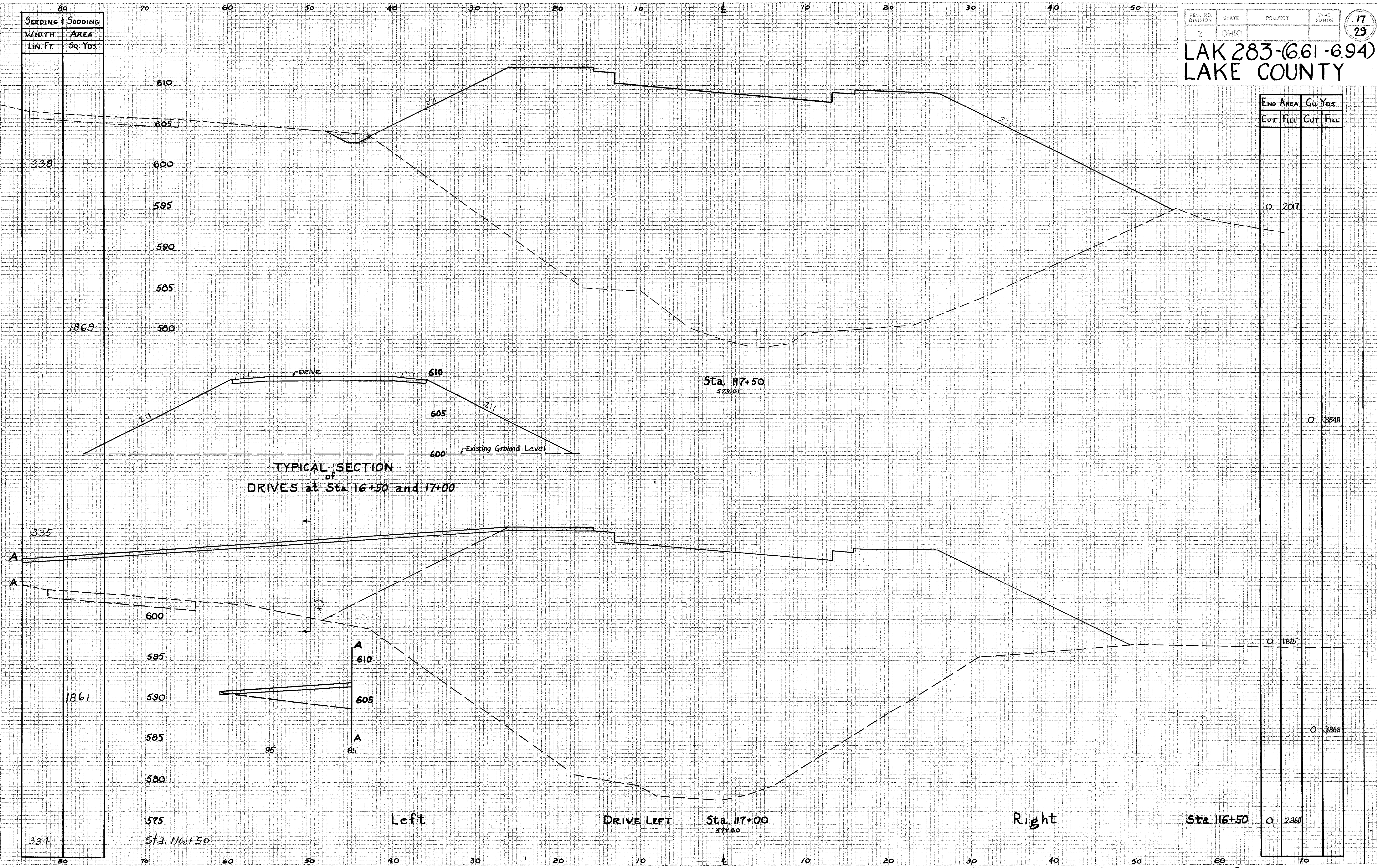
X-SECTIONS STA. 117+00 TO STA. 117+50
