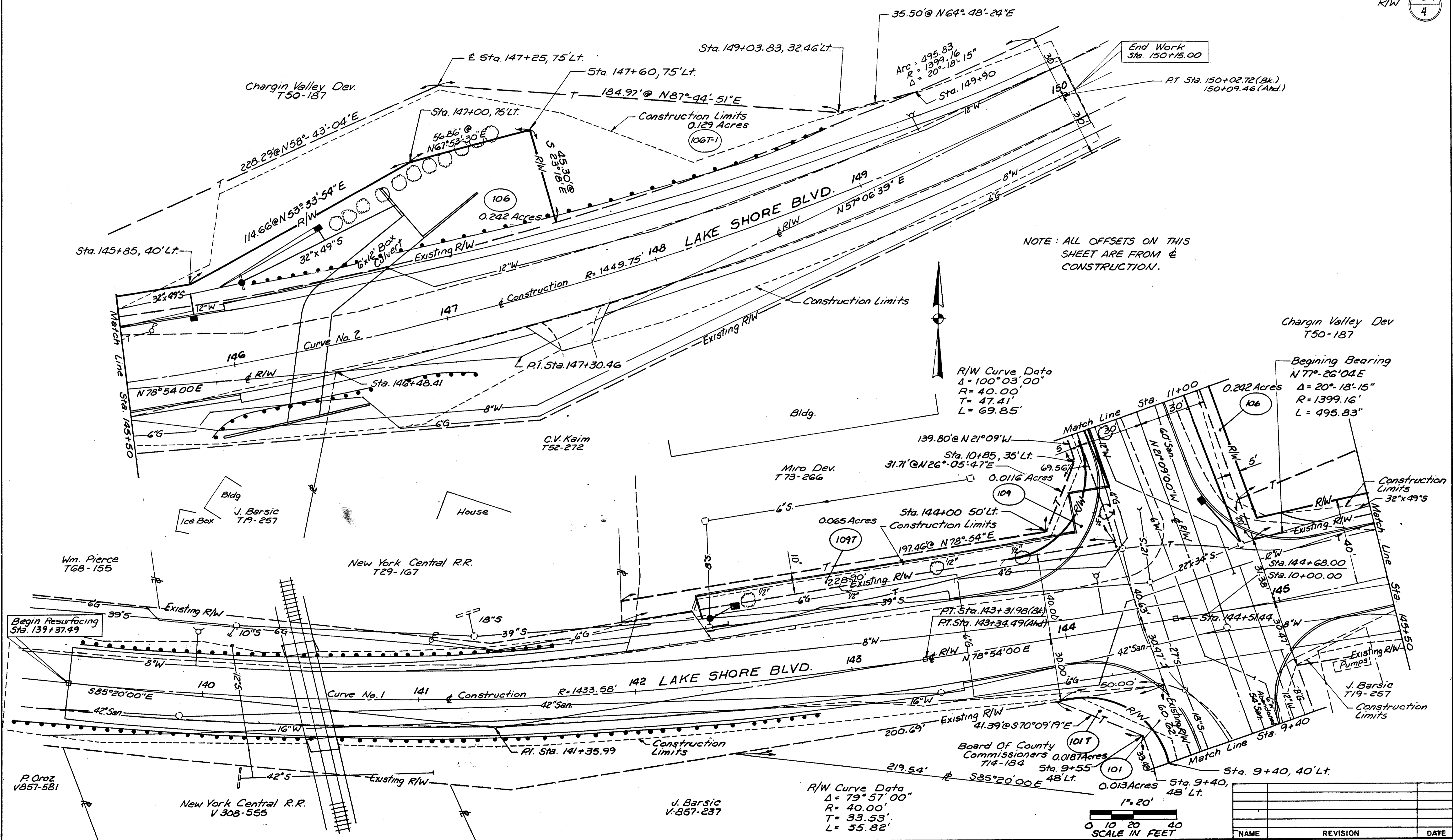
RIGHT OF WAY PLAN LAKE SHORE BLVD. S.R. 283 STA. 139+37 TO STA 150+15
